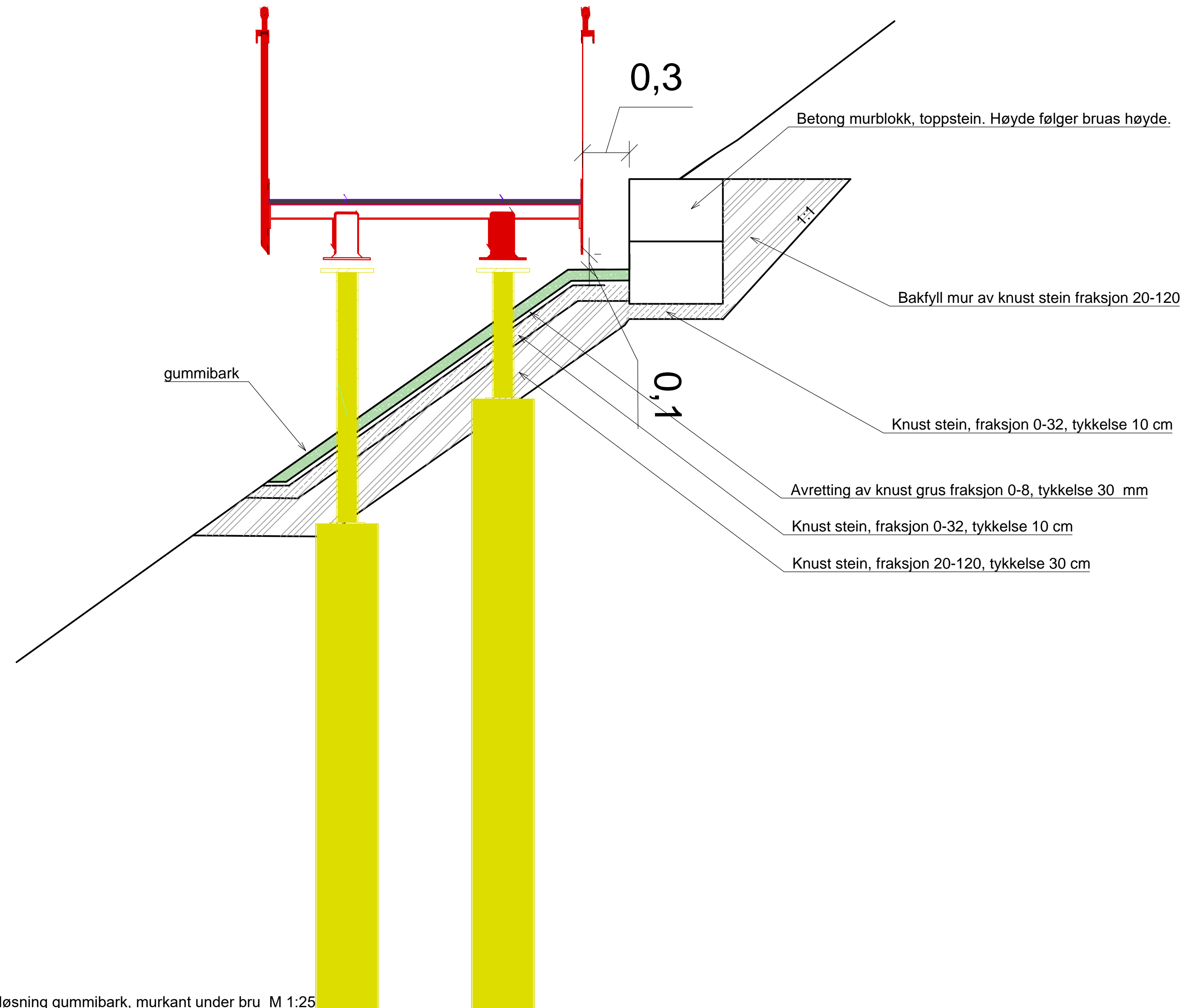
Snitt løsning gummibark, murkant under bru M 1:25
