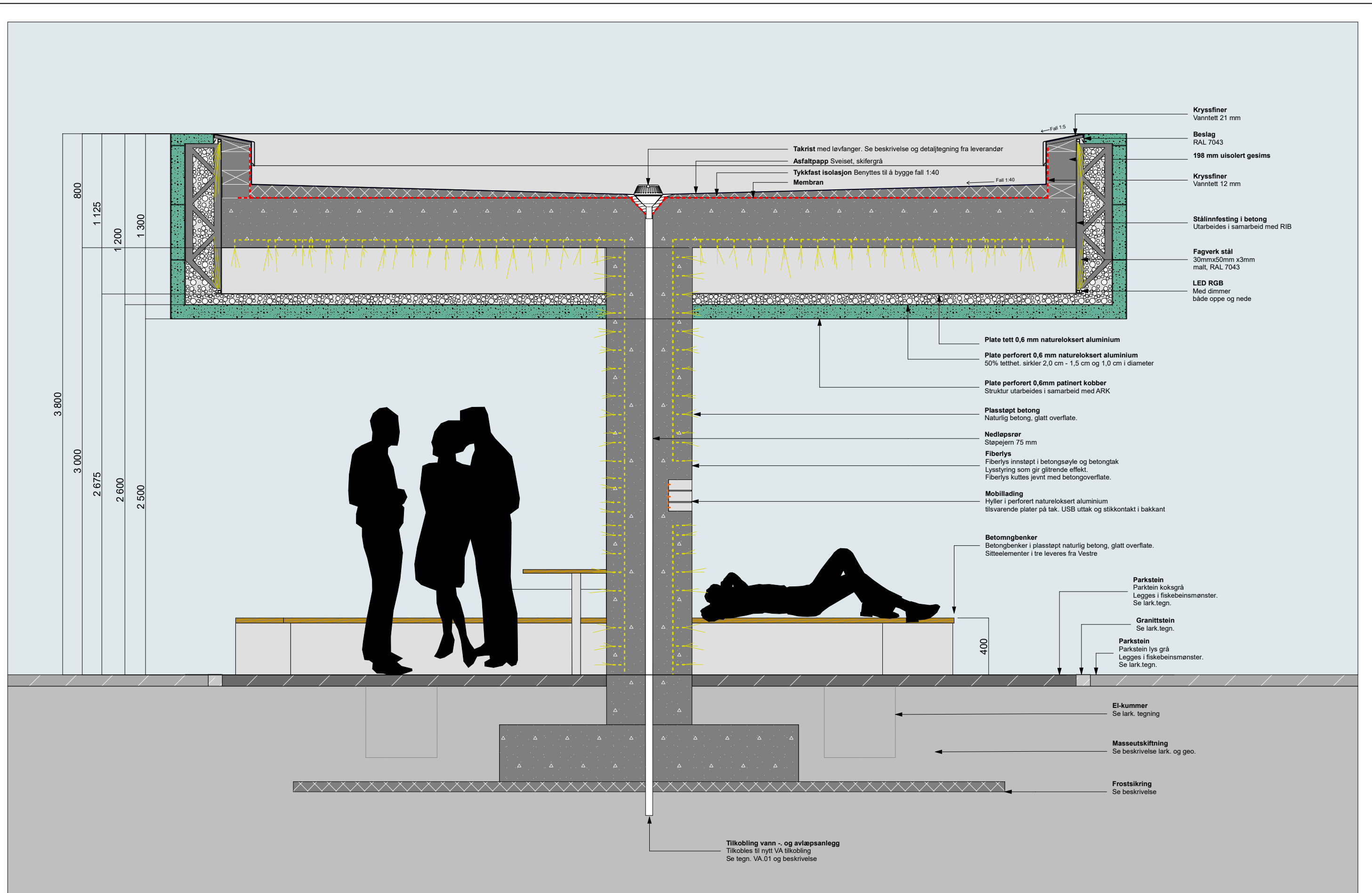
5172694 - A40-1 - Rismelparken - Anbudsgrunnlag - Parkpaviljong snitt A - 12.03.18 - 1:25
