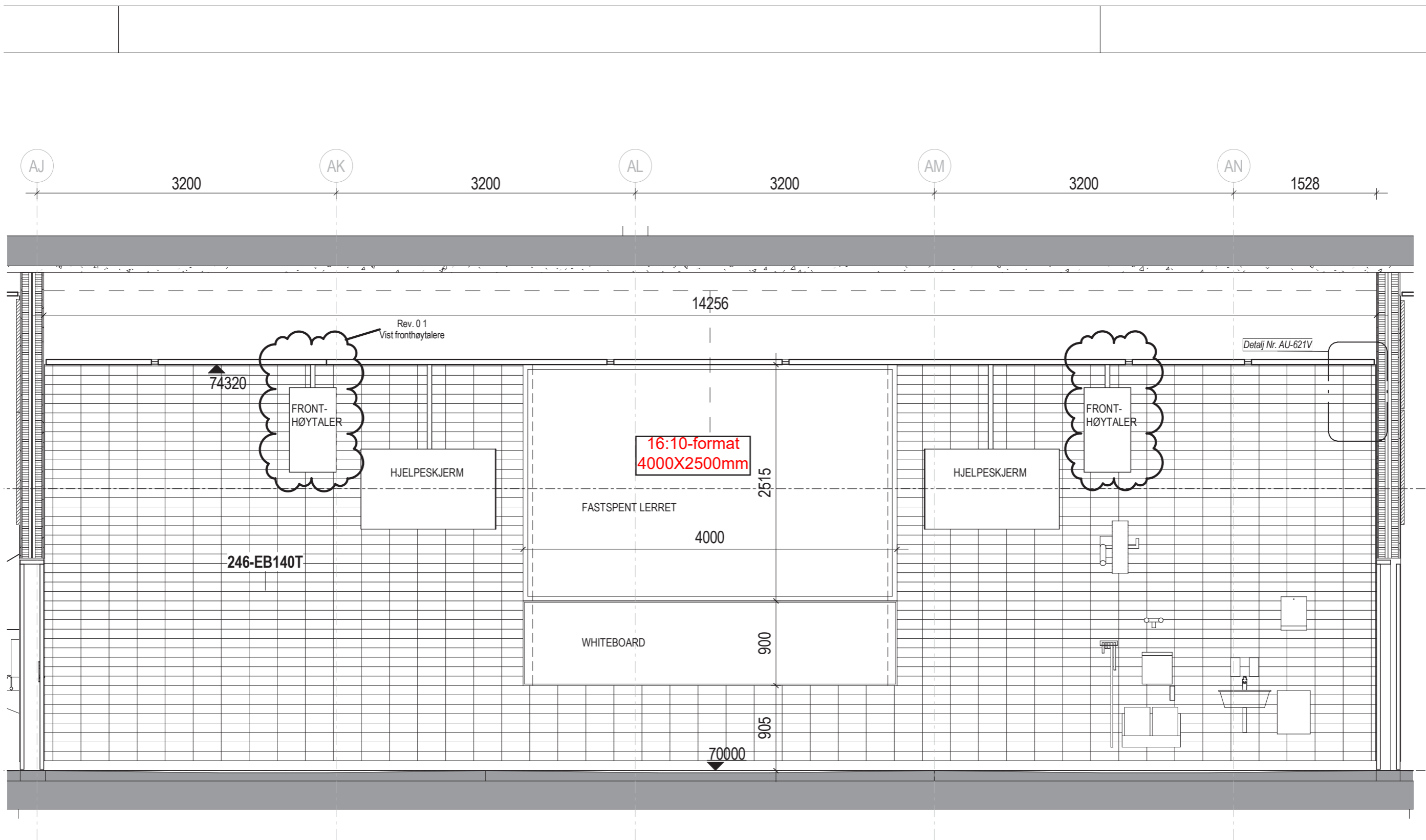
206.01.740 Auditorium Oppriss D Romskjema
