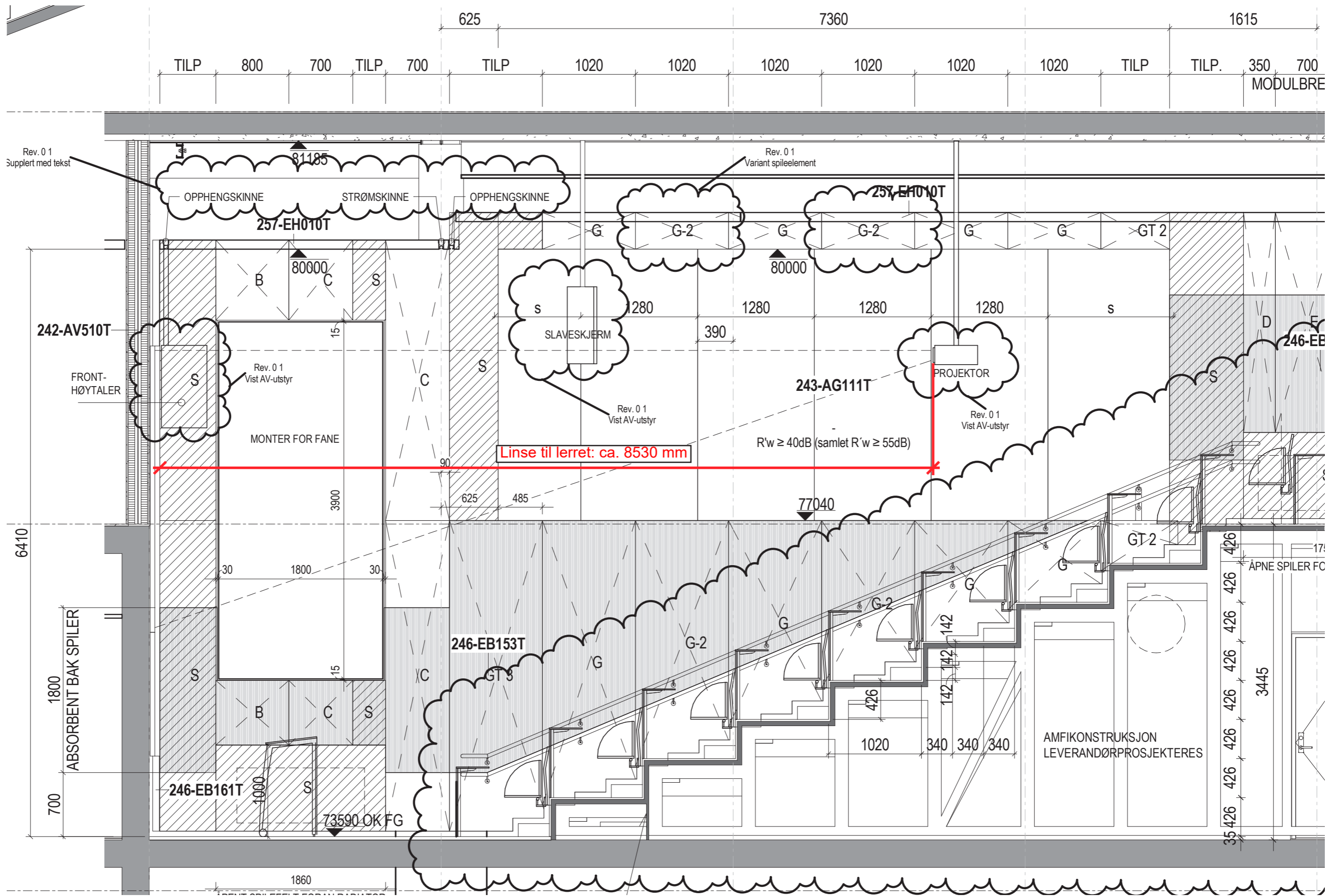
SNITT BYGG 154 - PLAN 01
