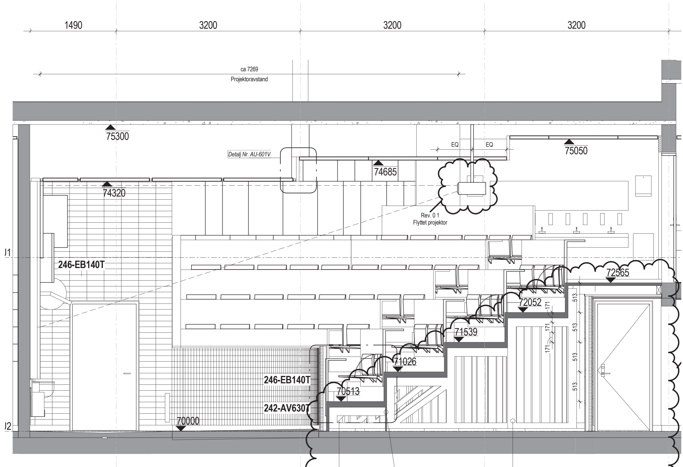
SNITT BYGG 153 - PLAN U2
