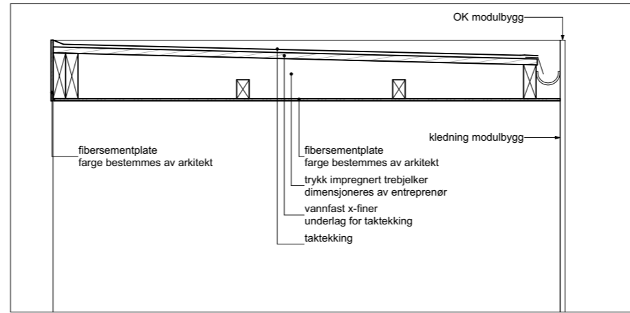
Snitt tak levegg 1:20
