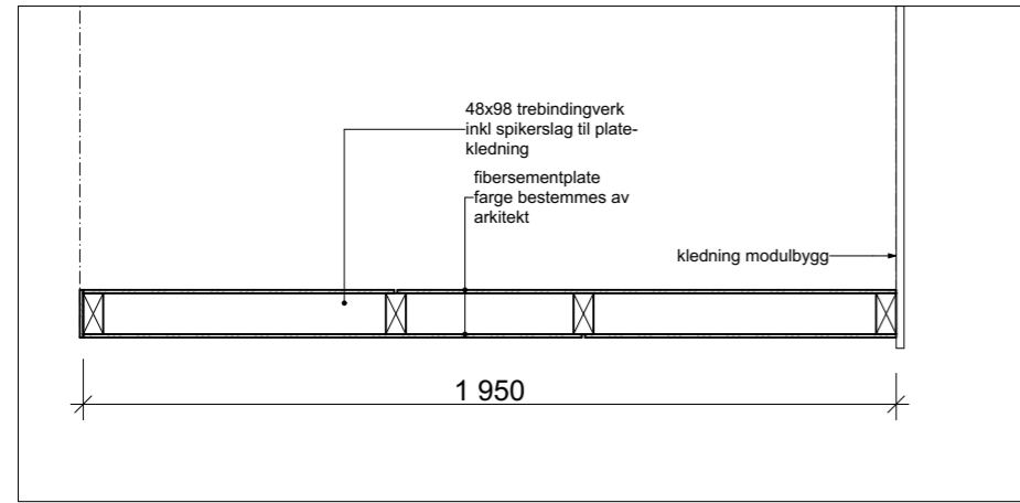
Planutsnitt levegg 1:20
