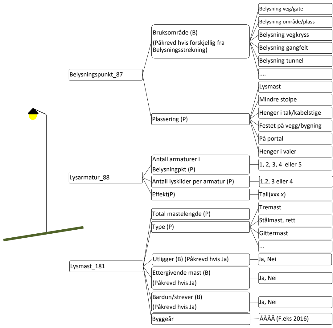
Figur 12. Eksempel på NVDB-objekter med påkrevde(P)og betingede(B) egenskaper (dette er en prinsippkisse)
