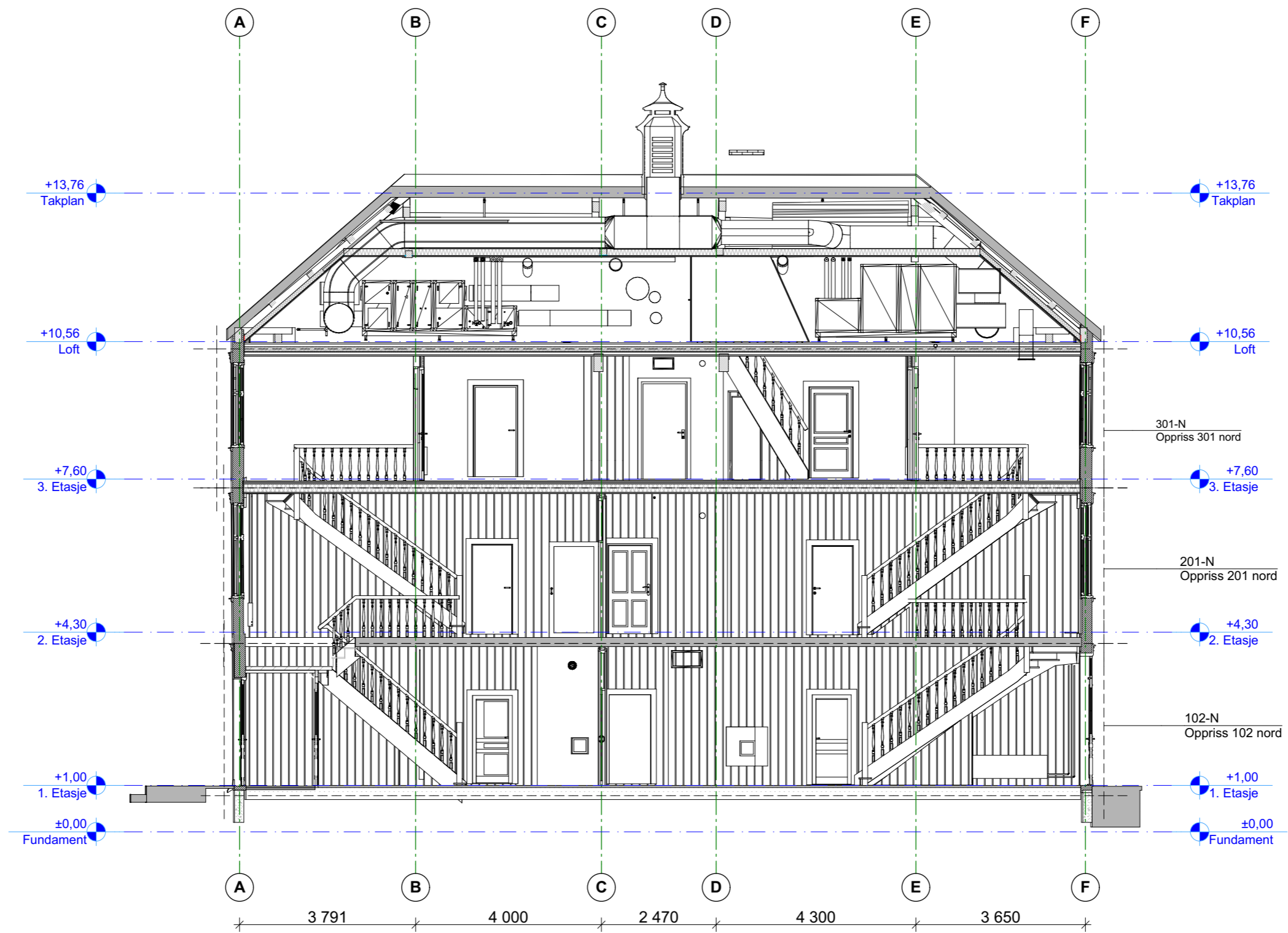
1:100 Snitt G
