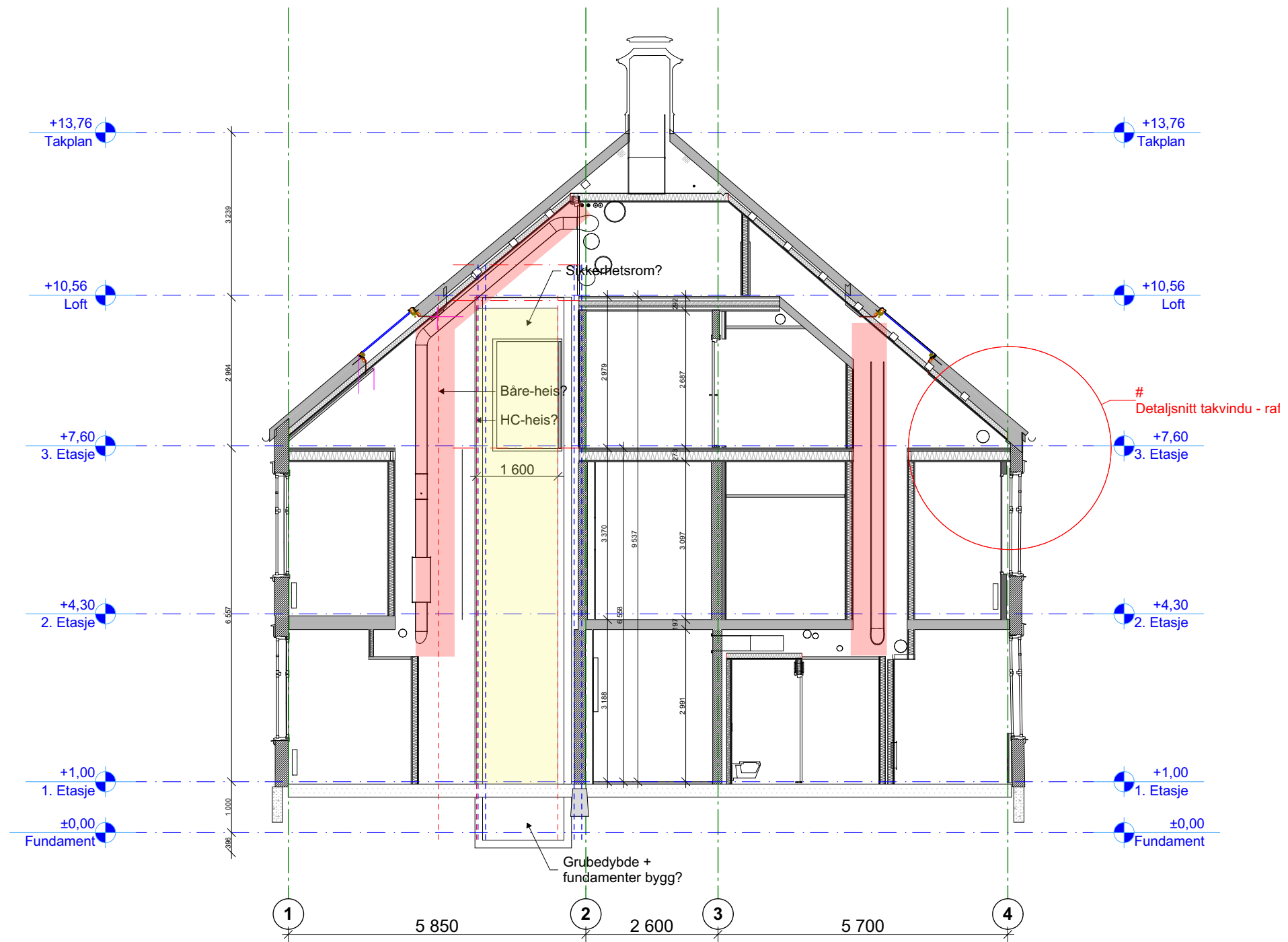
1:100 Snitt C
