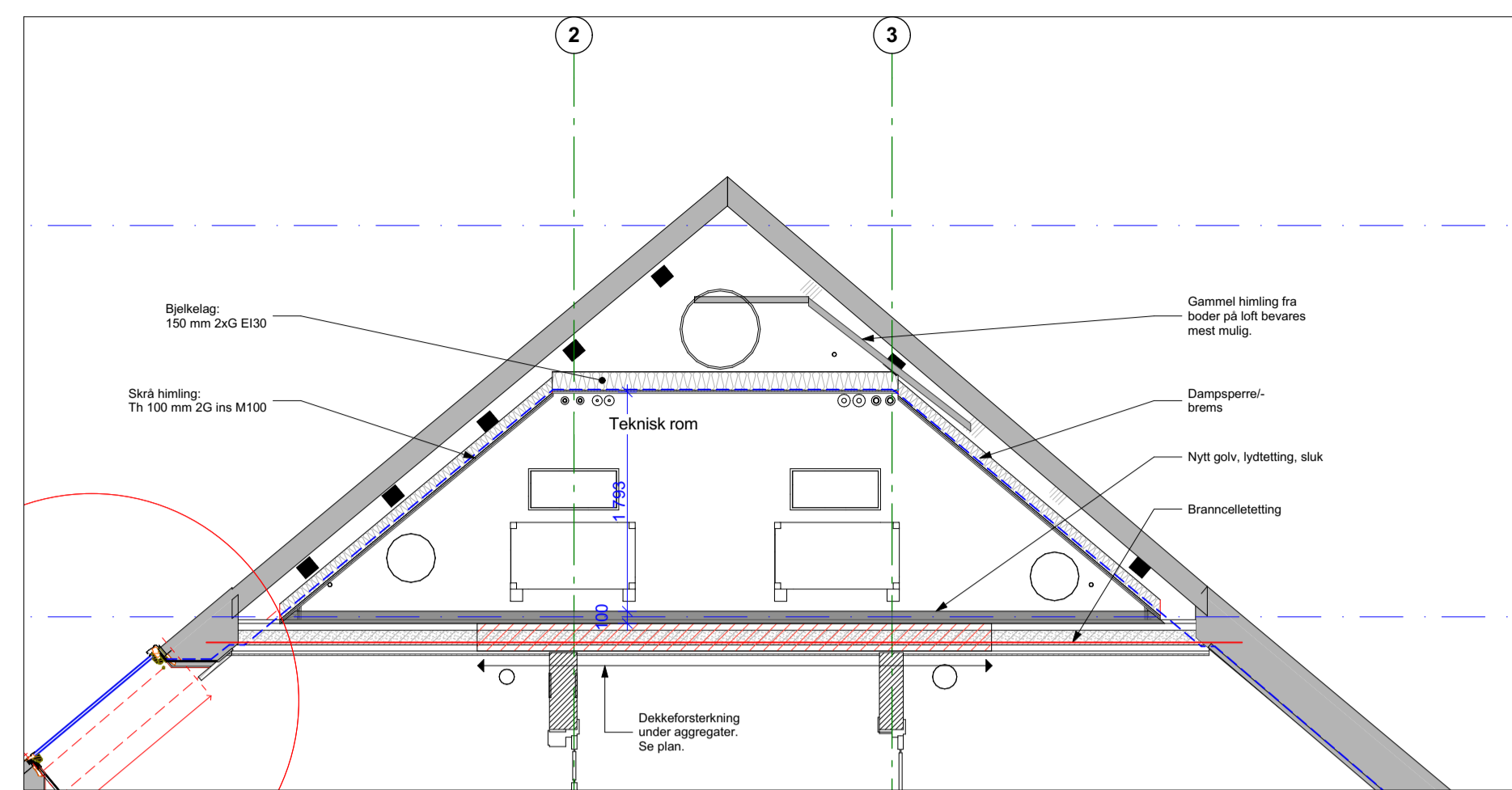
SNITT B, 1:50
