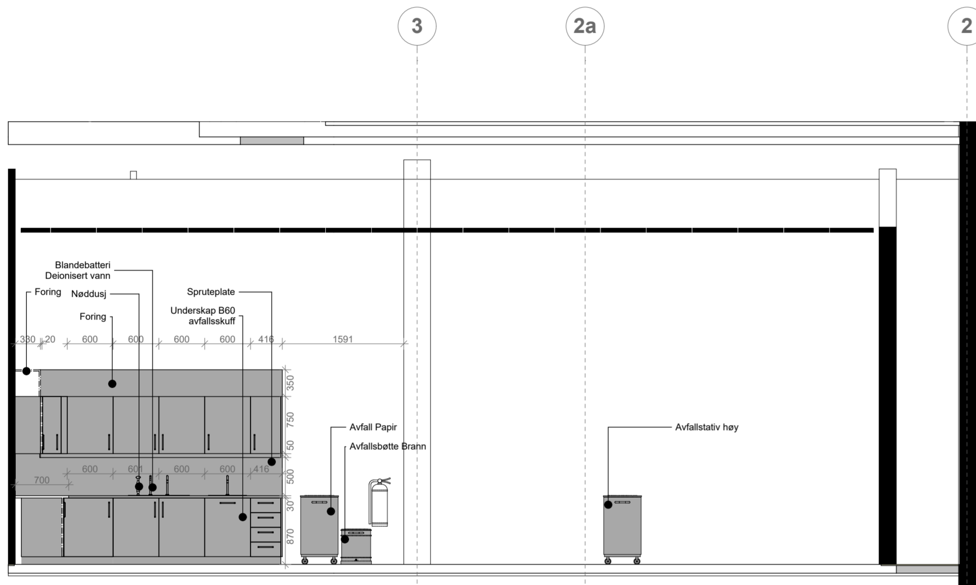
4 | 2 42 109A 04.01.013_Våtrom_Tekstil 1:50
