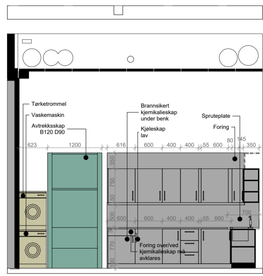
4 | 2 42 109B 04.01.013_Våtrom_Tekstil 1:50
