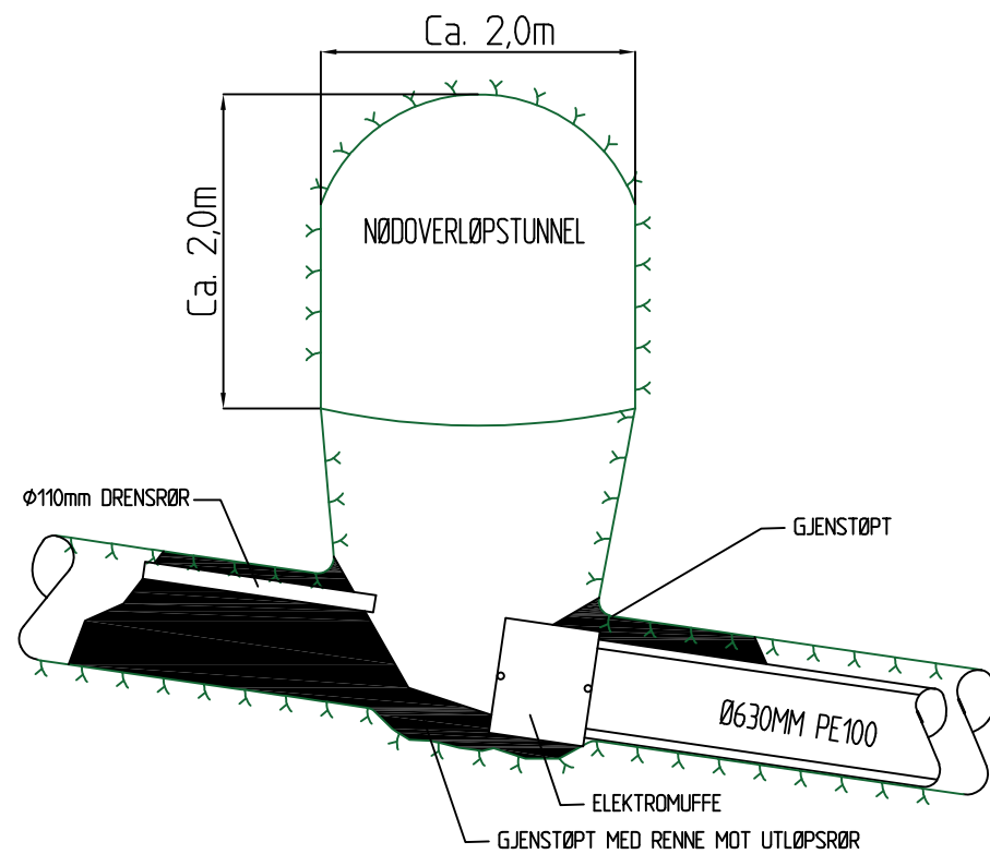
SITUASJON FERDIG TRUKKET RØR OG STØPT RENNE
