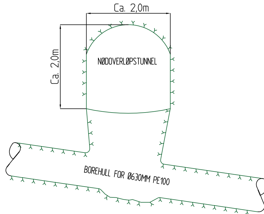
SITUASJON FJELL FJERNET NED TIL BOREHULL
