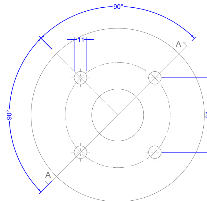
Spesiallaget monteringsplate til belysningsmodul A2 1:2
