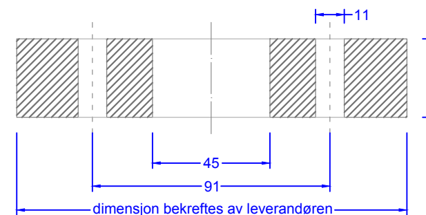
Snitt A 1:2
