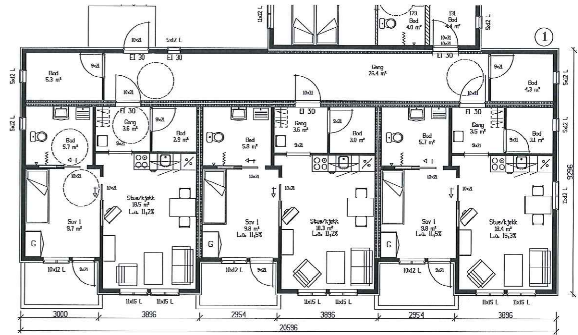
UTSNITT AV TILBYGG HOV.PLAN I MAL 1:100
