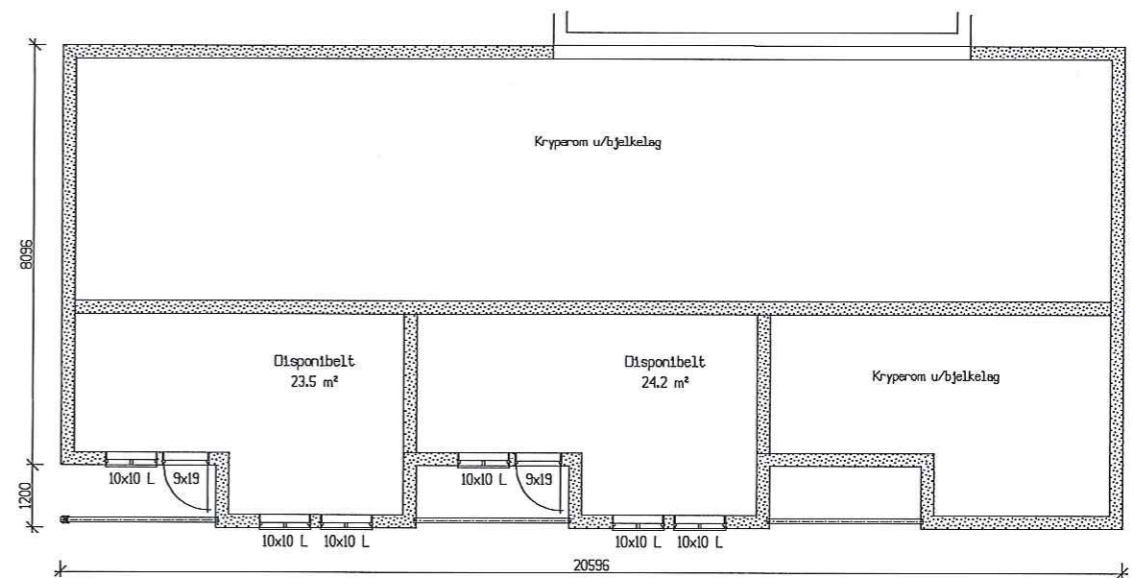
UTSNITT AV TILBYGG U.ETG I MAL 1:100
