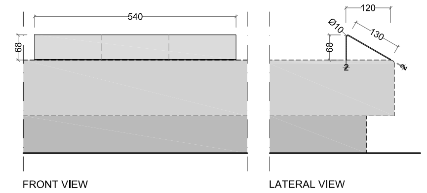
LH_T2-H130L540
