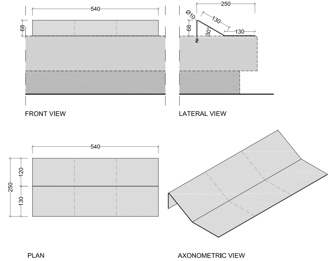
LH_T1-H260L540
