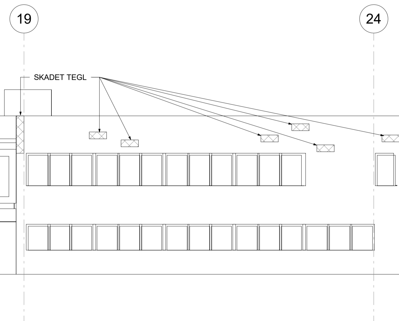
Fasade Øst - Akse 19-24 1 : 100
