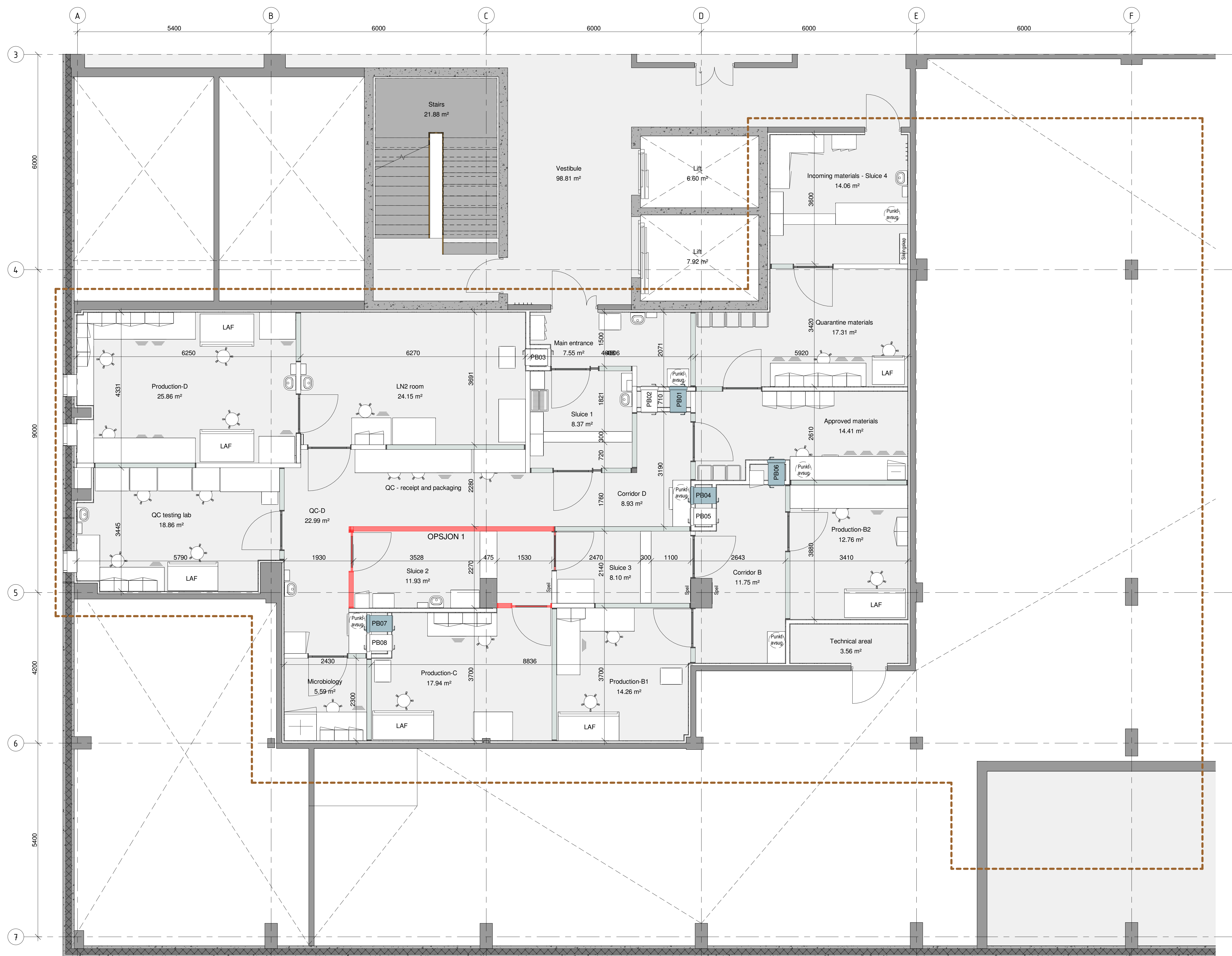
Plan 1M - Byggleveranse 1 : 50
