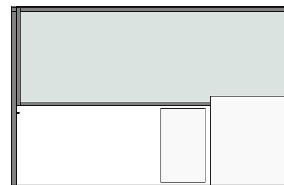
Production-C - vegg B 1 : 50
