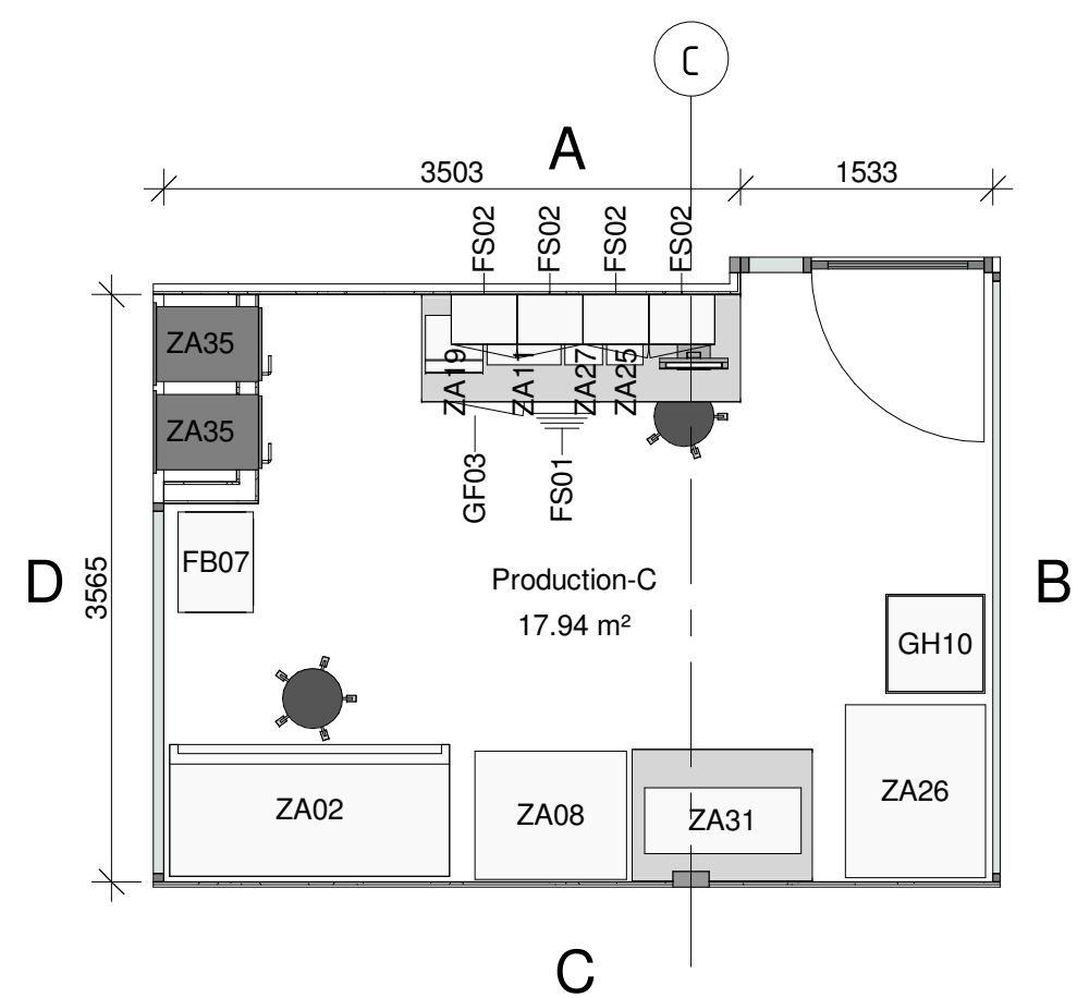
Plan Production-C 1 : 50
