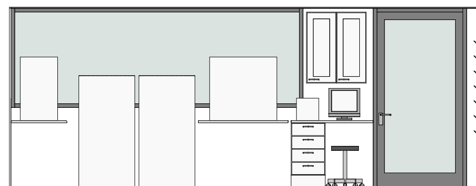
LN2 room - vegg C 1 : 50
