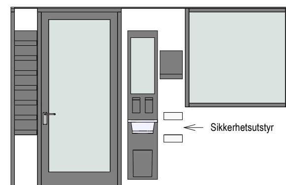
LN2 room - vegg D 1 : 50
