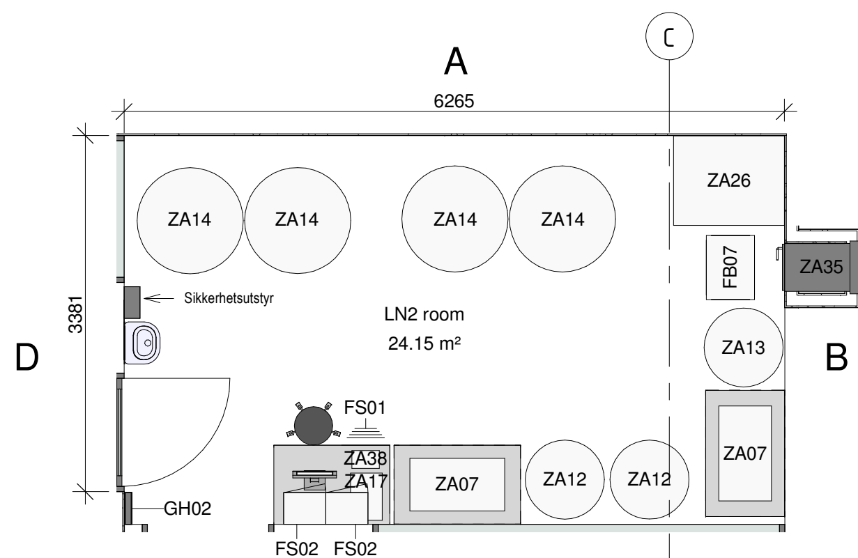
Plan LN2 room 1 : 50
