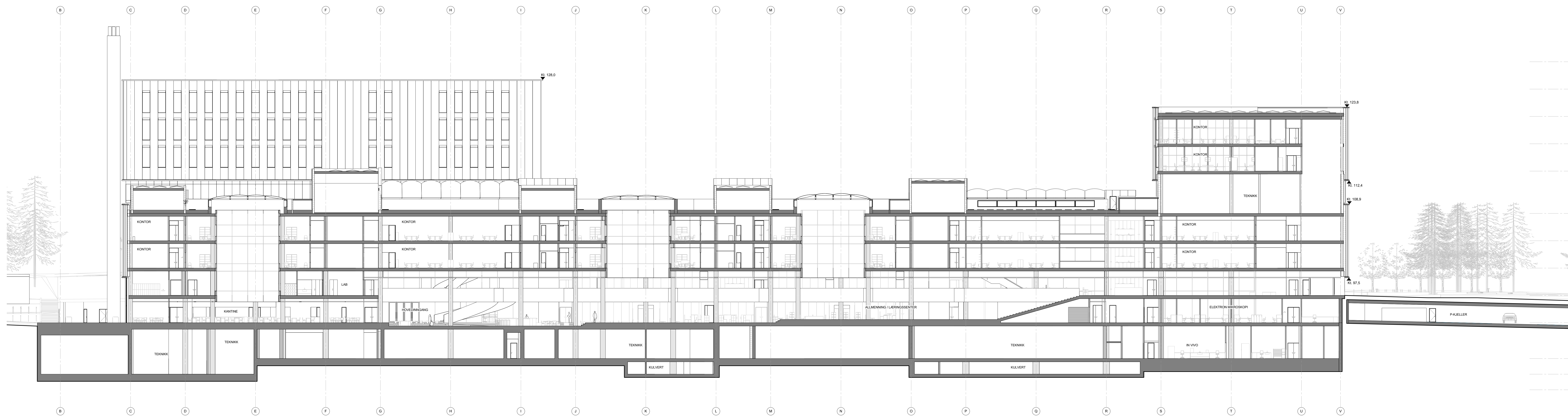
Snitt A-A
