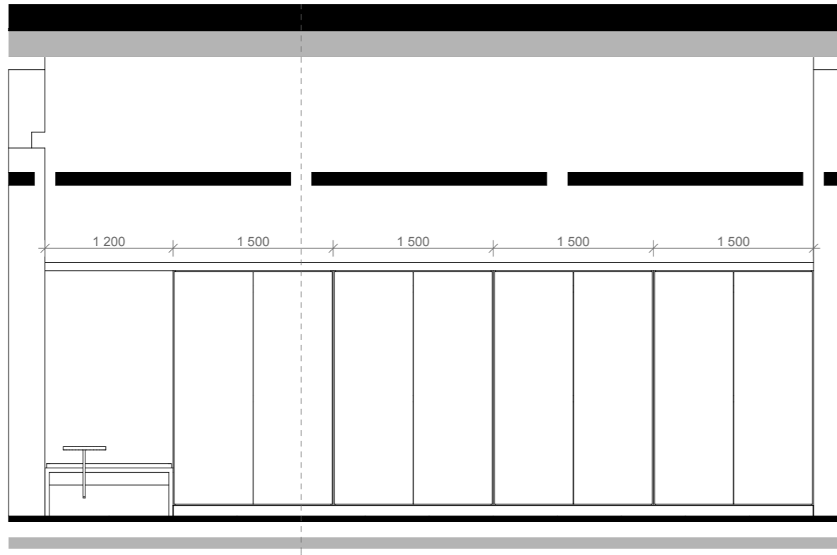
OPPRISS 05 | 2 42 121 1:50
