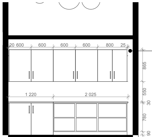
OPPRISS 05 | 2 42 113 1:50
