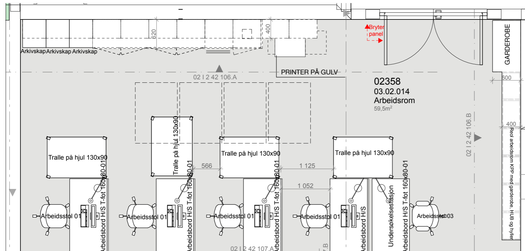
PLAN 1:50
