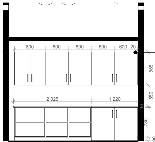
OPPRISS 05 | 2 42 115 1:50
