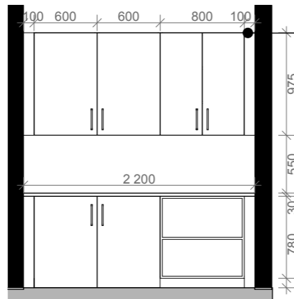
OPPRISS 04 | 2 42 153 1:50
