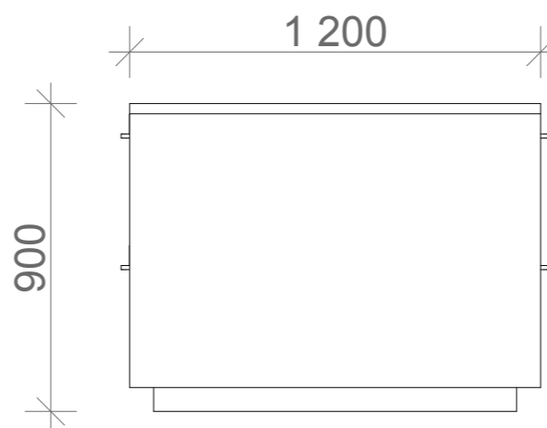
OPPRISS B-B 1:20
