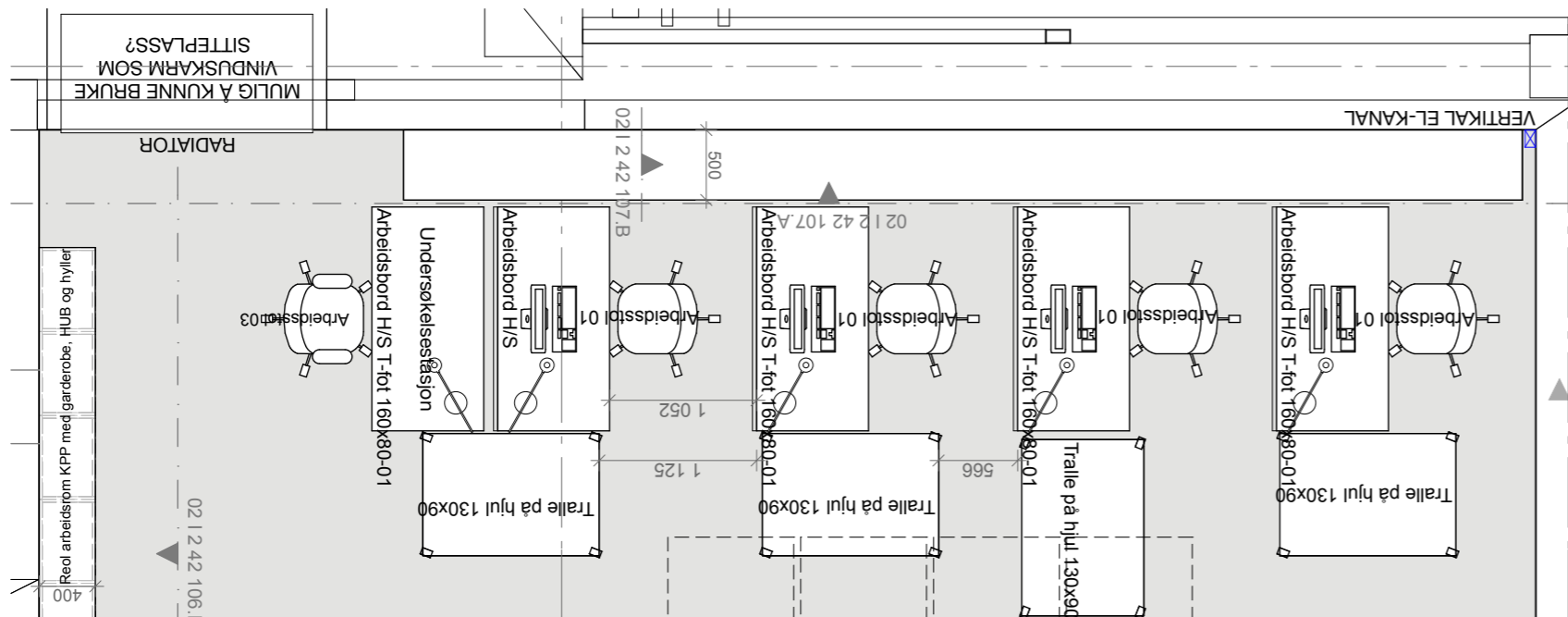
PLAN 1:50
