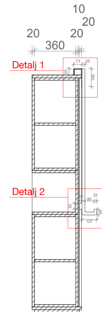
SNITT C-C 1:20
