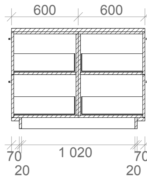
SNITT C-C 1:20
