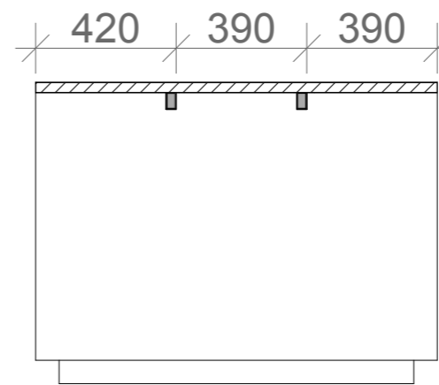
SNITT C-C 1:20
