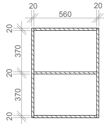
SNITT B-B 1:20
