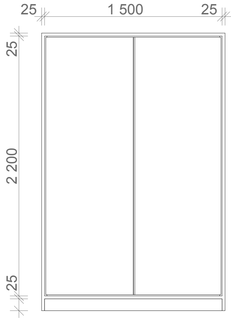
OPPRISS A-A 1:20
