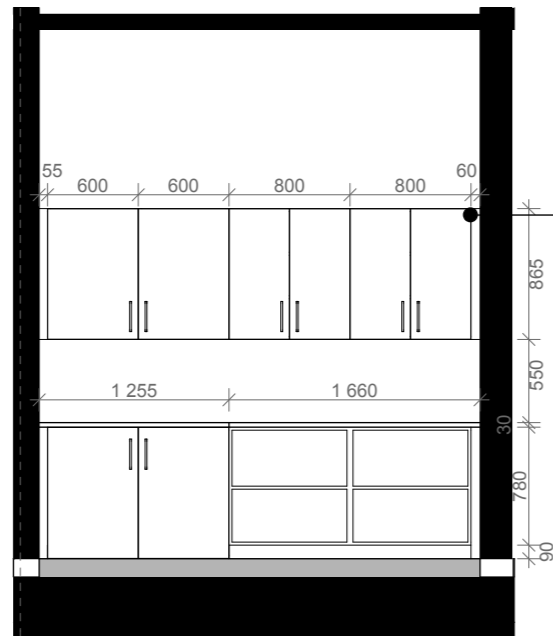
OPPRISS 02 | 2 42 123 1:50
