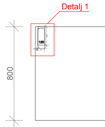
OPPRISS A-A 1:20
