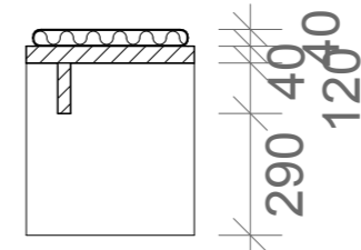
SNITT B-B 1:20
