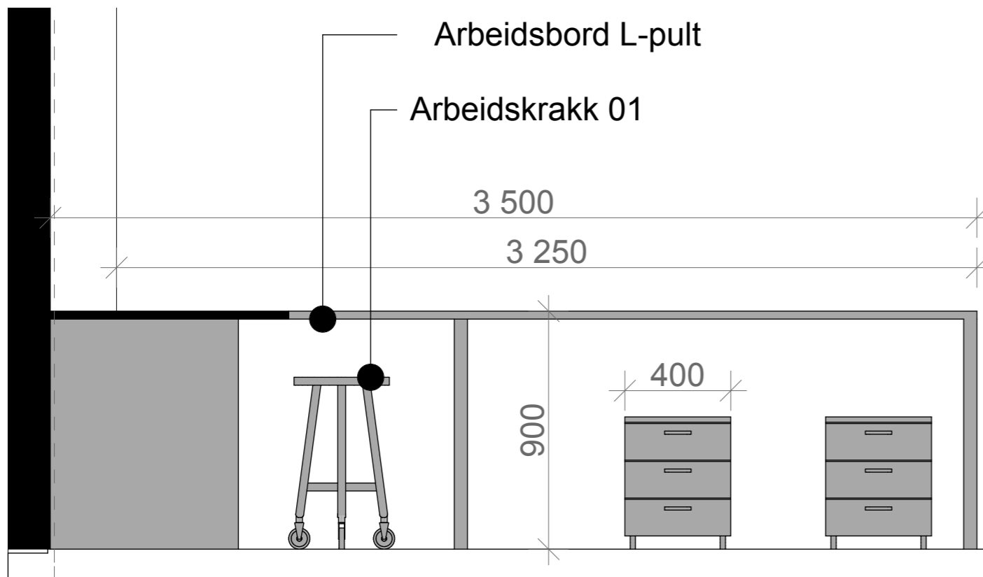
FRONT OPPRISS 1:20
