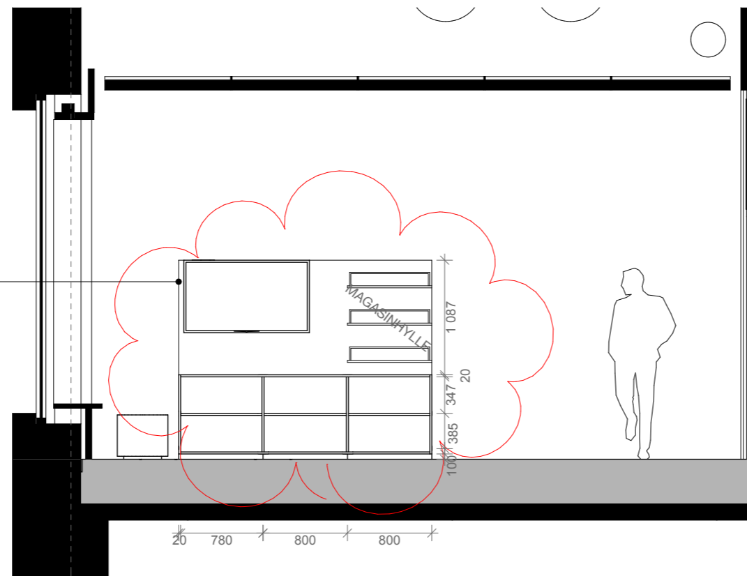
OPPRISS 02 | 2 42 101 1:50
