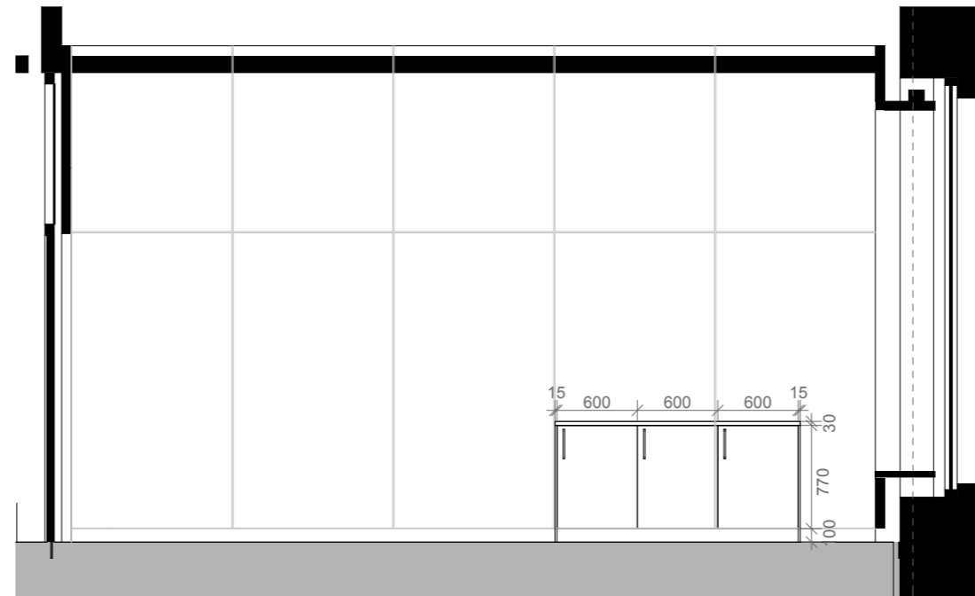
OPPRISS 02 | 2 42 124.B 1:50
