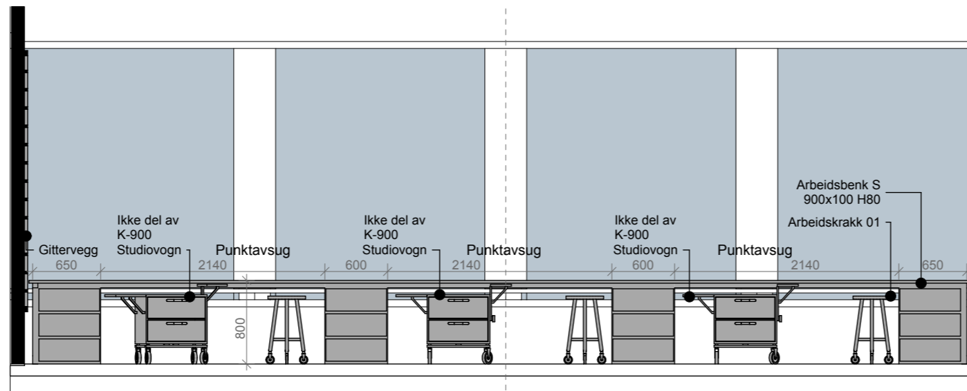
FRONT OPPRISS 1:50
