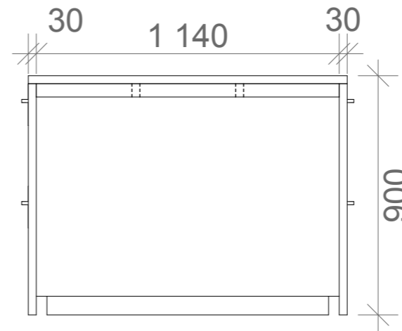
OPPRISS B-B 1:20
