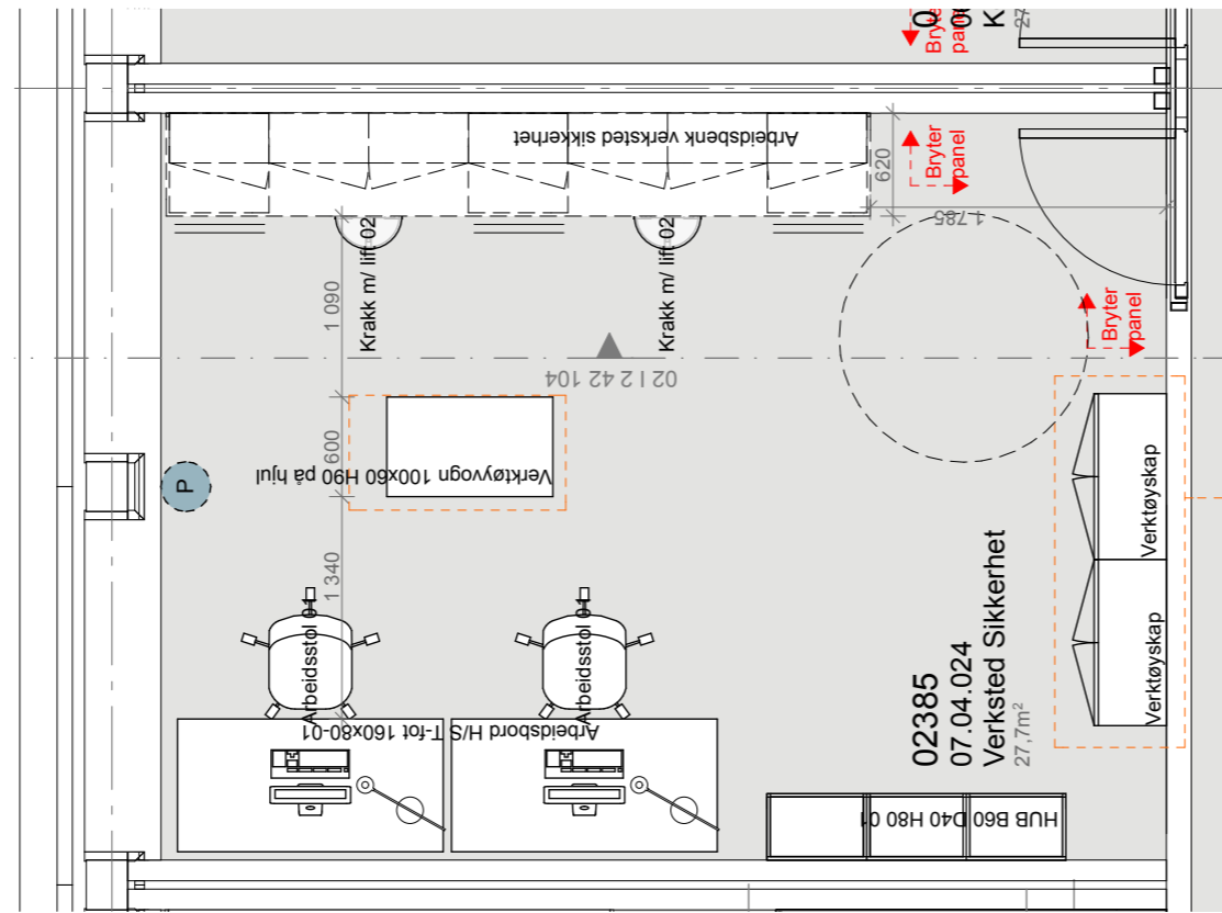
PLAN 1:50
