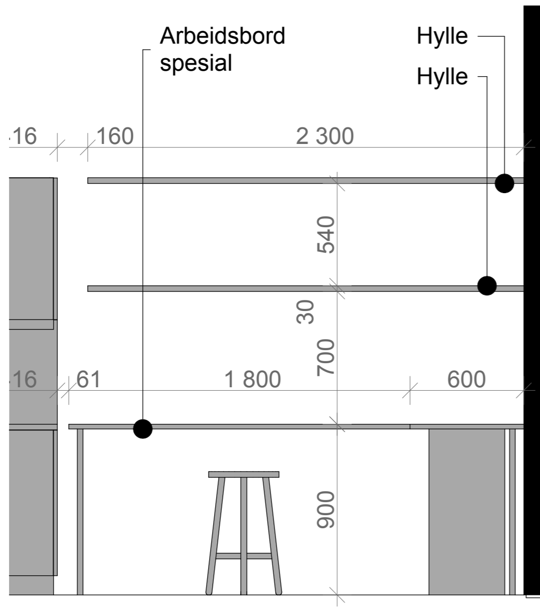
FRONT OPPRISS 1:20
