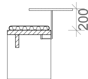
Prinsipp med fastmontert bord Ø400
