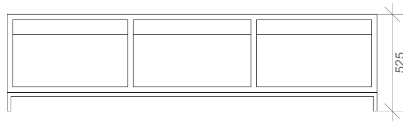
OPPRISS A-A 1:20
