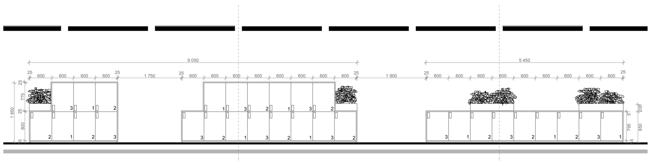
OPPRISS 05 | 2 42 107.A 1:50
