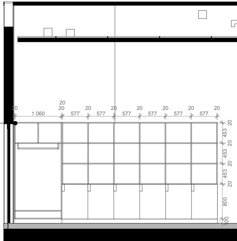
OPPRISS 02 | 2 42 106.B 1:50
