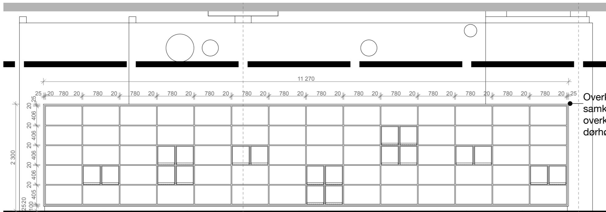
OPPRISS 05 | 2 42 117 1:50
