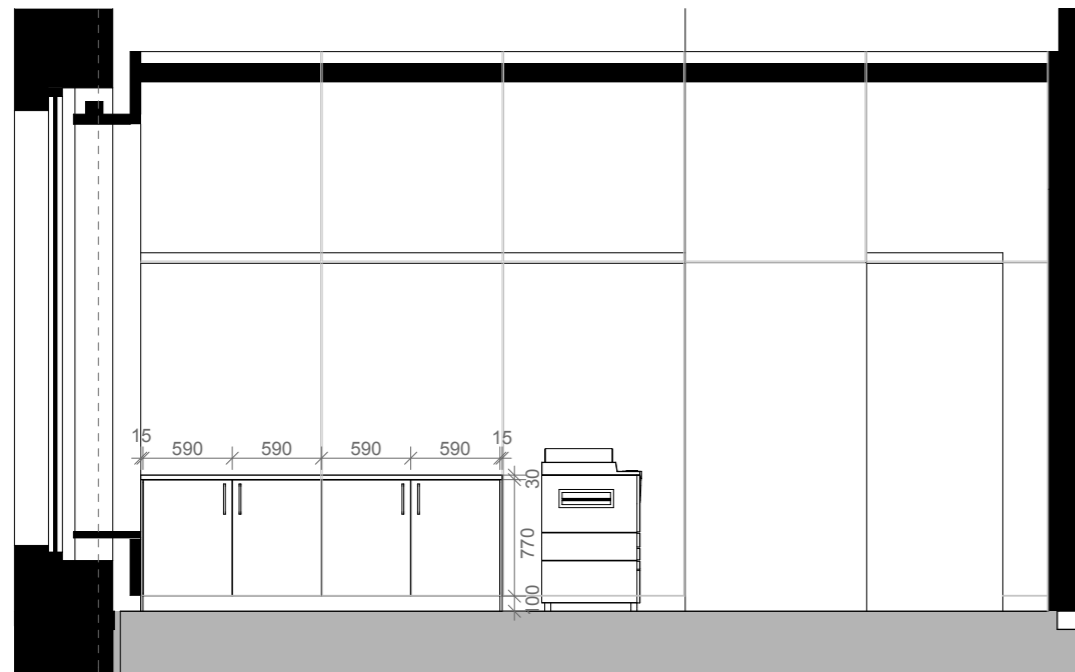
OPPRISS 02 | 2 42 124.A 1:50
