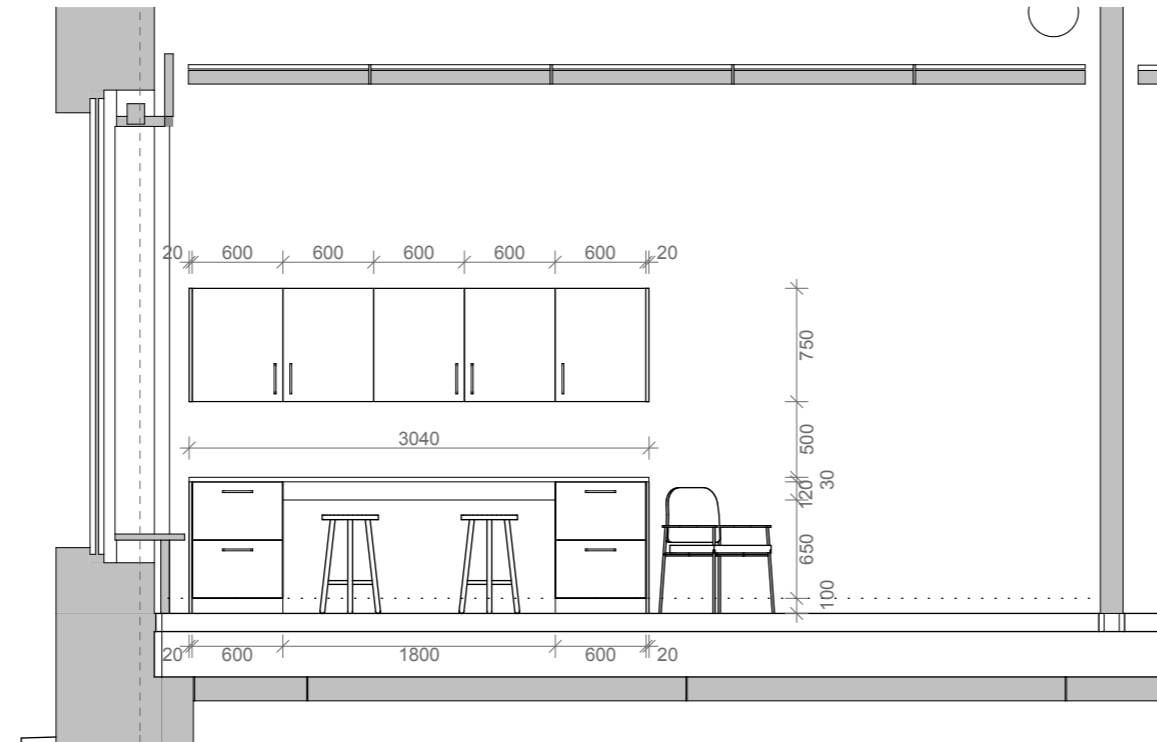
OPPRISS 02 | 2 42 105 1:50
