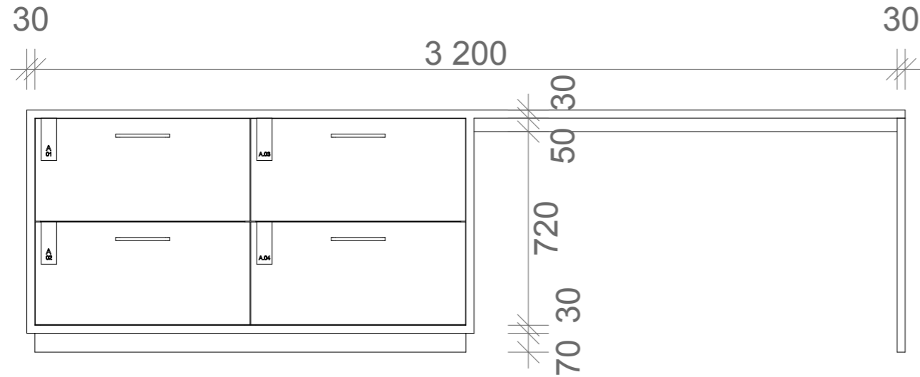
OPPRISS A-A 1:20
