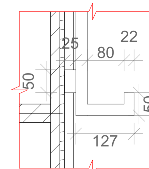
DETALJ 2 1:5
