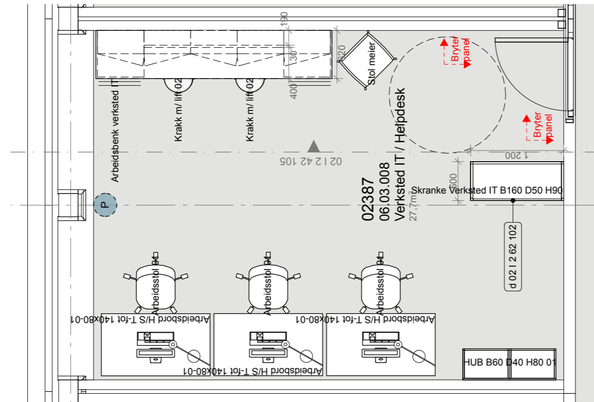
PLAN 1:50
