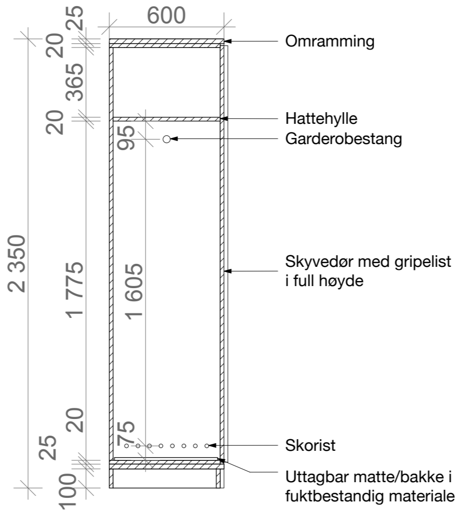
PRINSIPP SNITT 1:20
