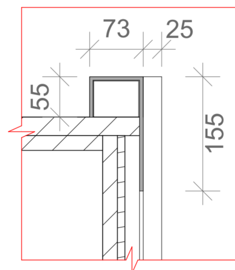
DETALJ 1 1:5
