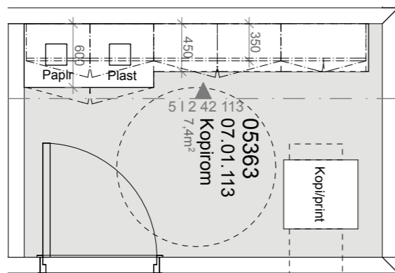
PLAN 1:50
