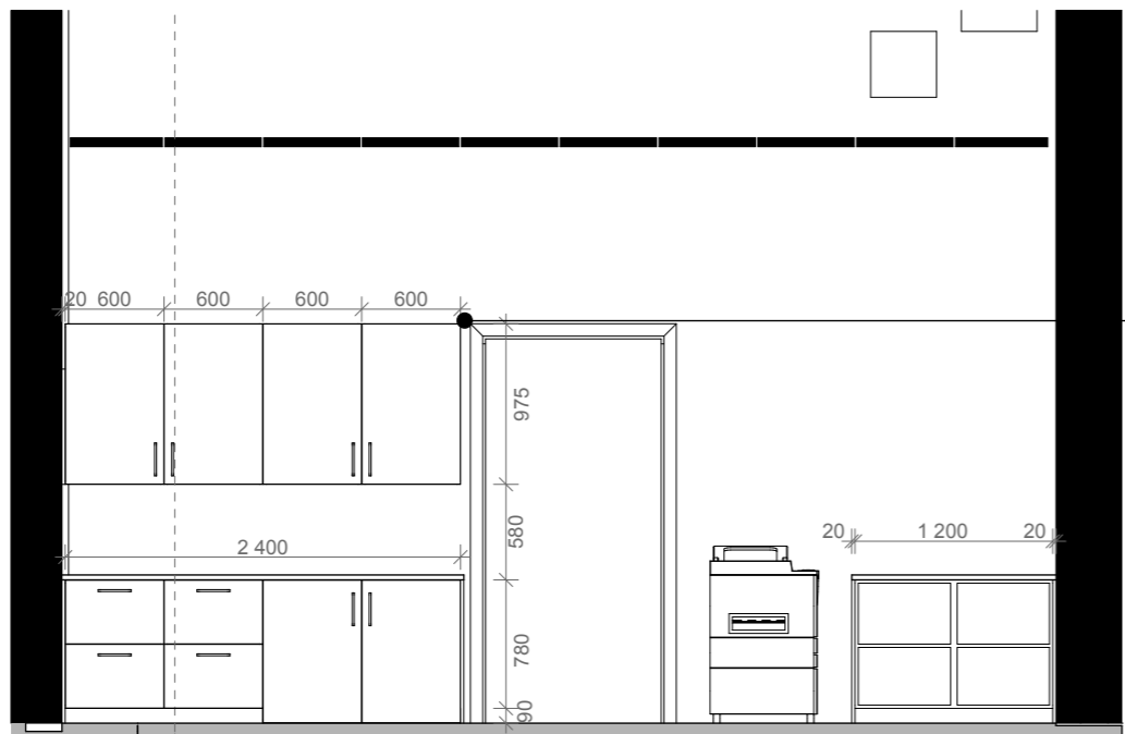
OPPRISS 03 | 2 42 152 1:50
