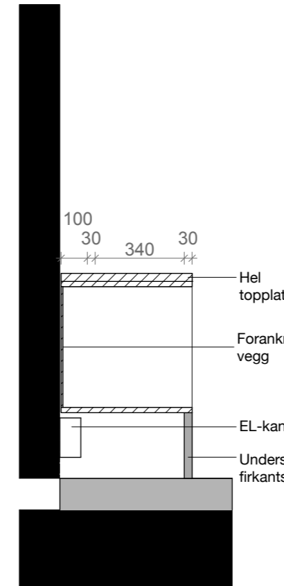
SNITT 02 | 2 42 107.B 1:20
