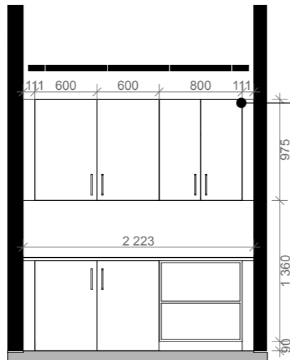
OPPRISS 03 | 2 42 153 1:50
