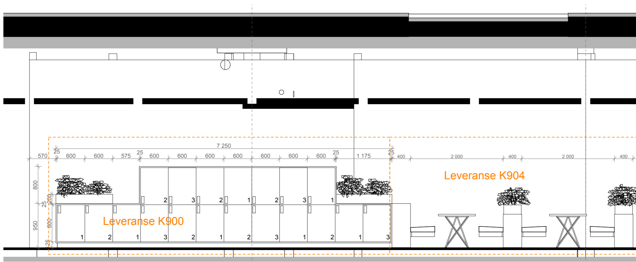
OPPRISS 05 | 2 42 109 1:50
