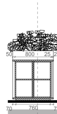
SNITT 05 | 2 42 110.C 1:50
