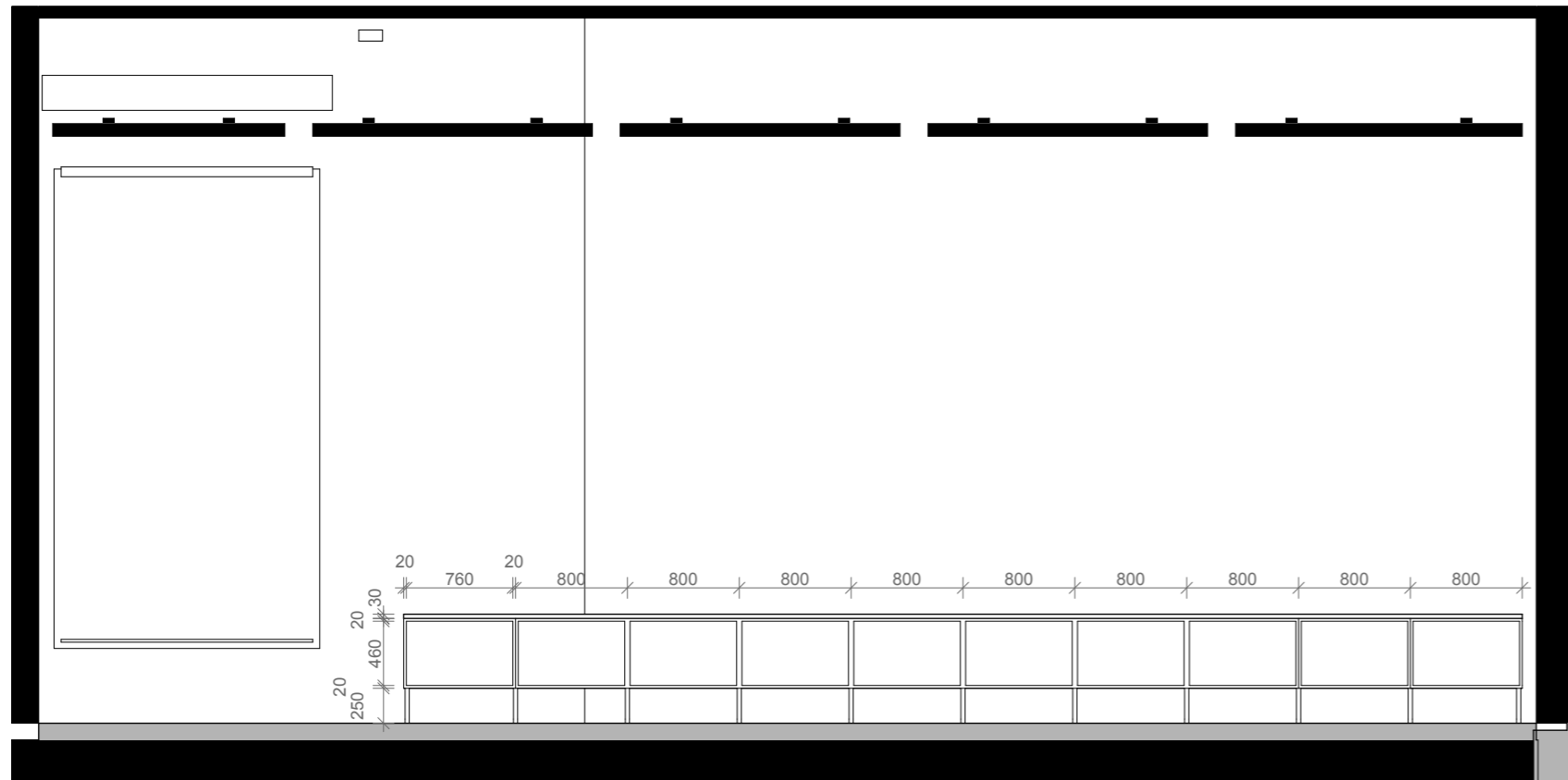
OPPRISS 02 | 2 42 107.A 1:50
