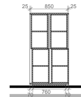
SNITT 05 I 2 42 112.D 1:50
