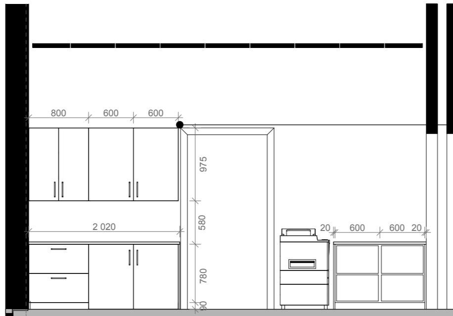
OPPRISS 04 | 2 42 152 1:50
