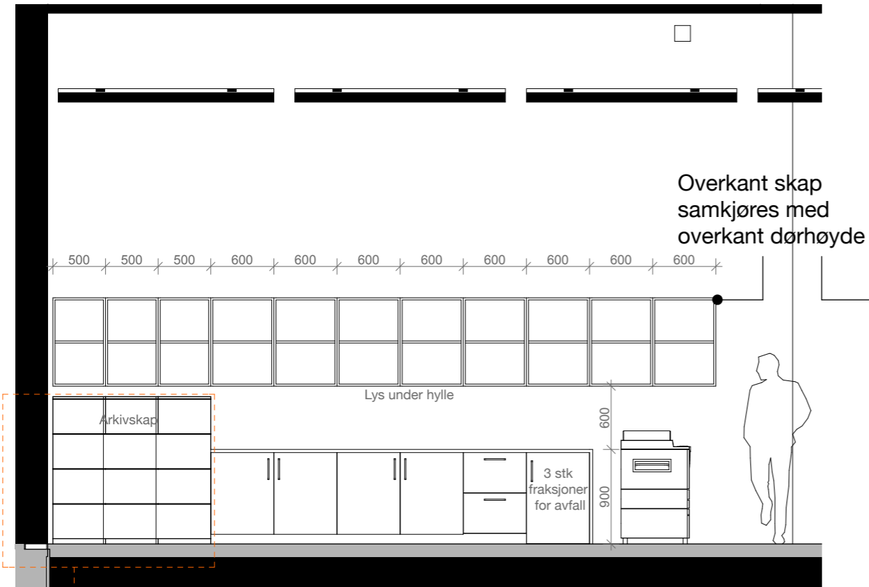
OPPRISS 02 | 2 42 106.A 1:50
