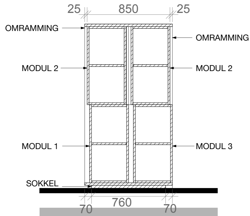
PRINSIPP SNITT 1:20
