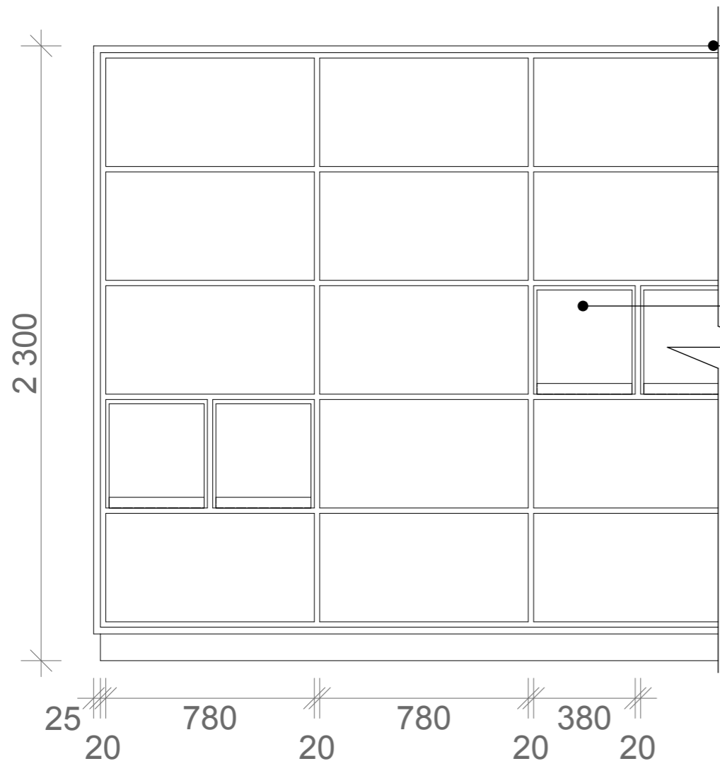
OPPRISS A-A 1:20
