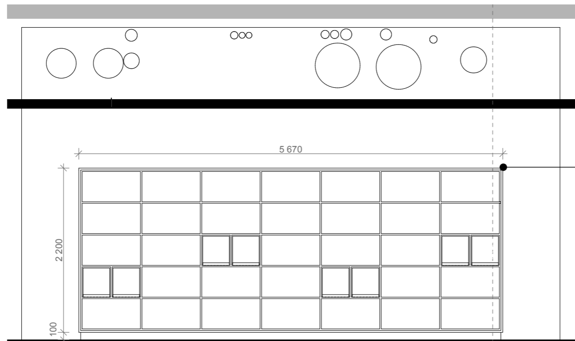
OPPRISS 05 | 2 42 102 1:50
