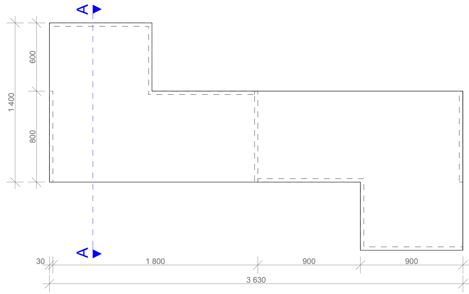
PLAN 1:20
