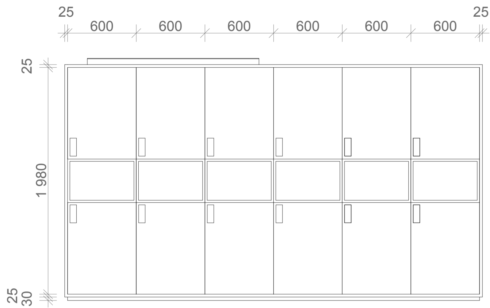
OPPRISS A-A 1:20
