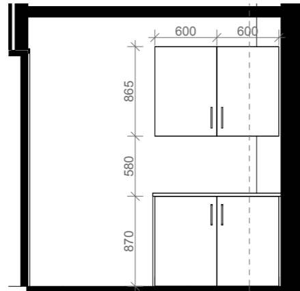
OPPRISS 05 I 2 42 114.A 1:50
