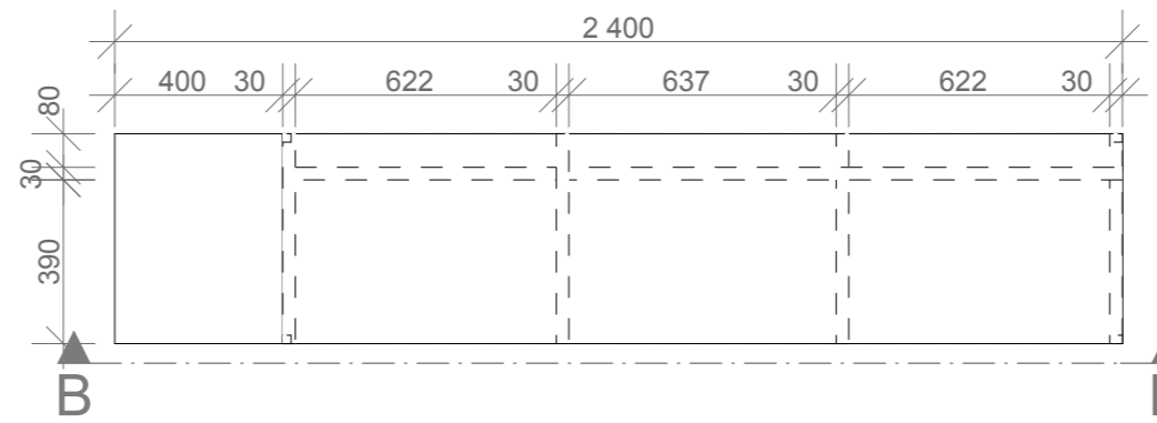
PLAN 1:20 HYLLE MIDTMODUL
