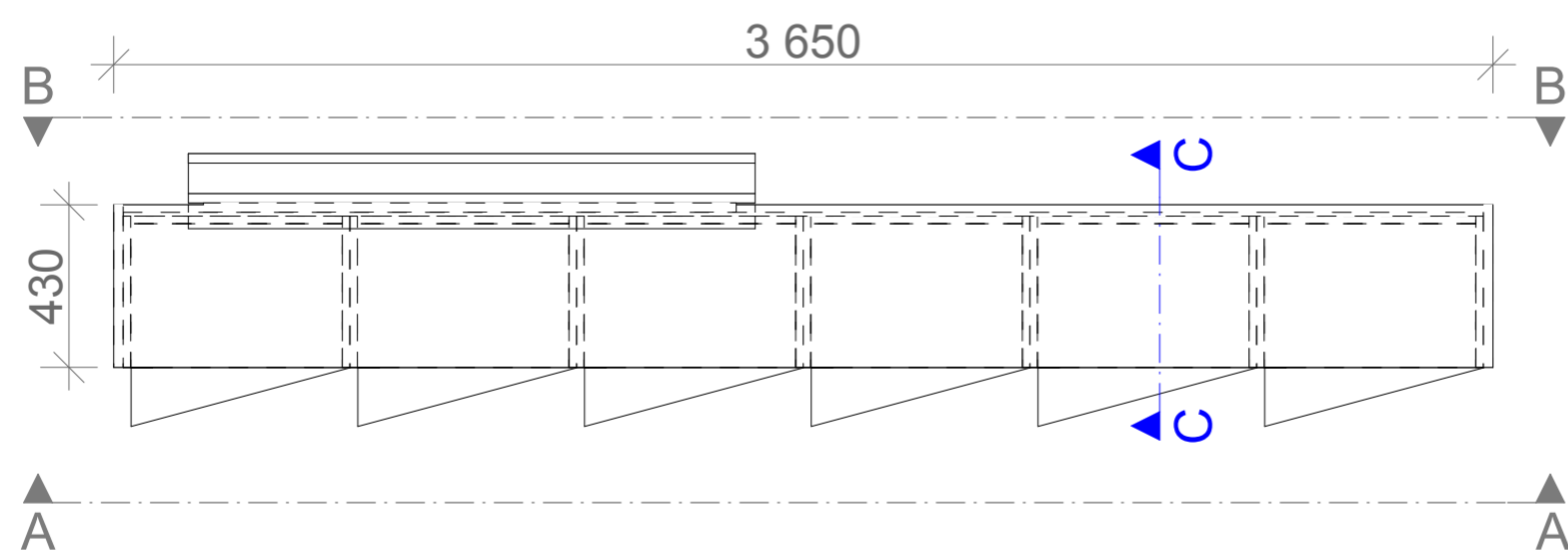
PLAN 1:20
