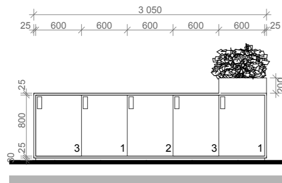
OPPRISS 05 | 2 42 110.A 1:50
