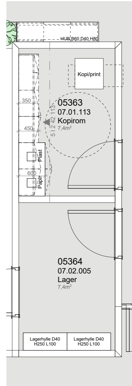
PLAN 1:50
