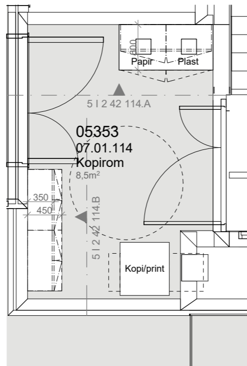
PLAN 1:50
