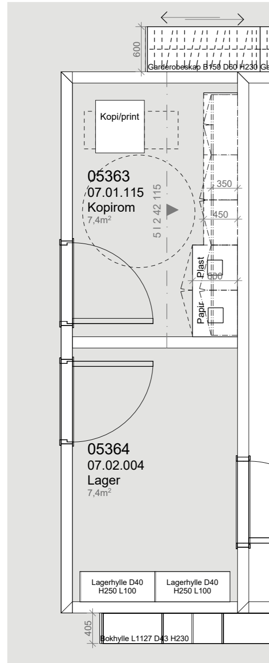
PLAN 1:50
