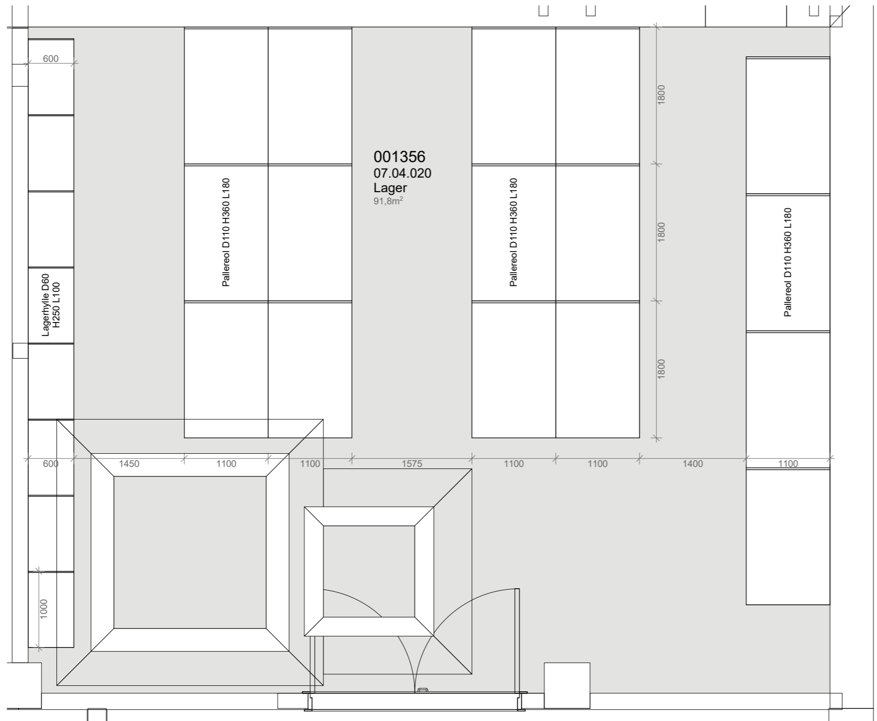
PLAN 1:50
