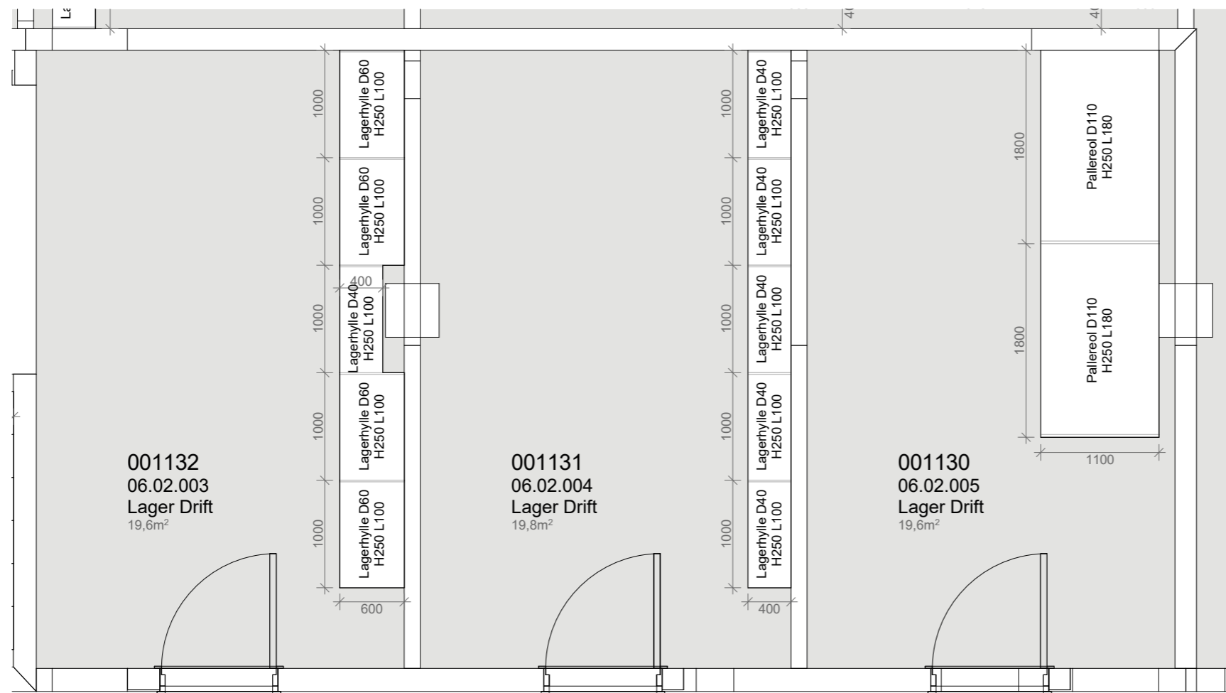
PLAN 1:50
