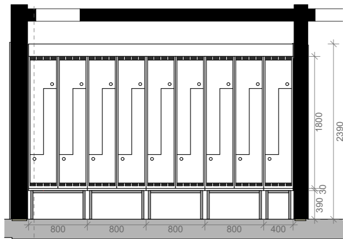
OPPRISS 001 | 2 63 103.A 1:50
