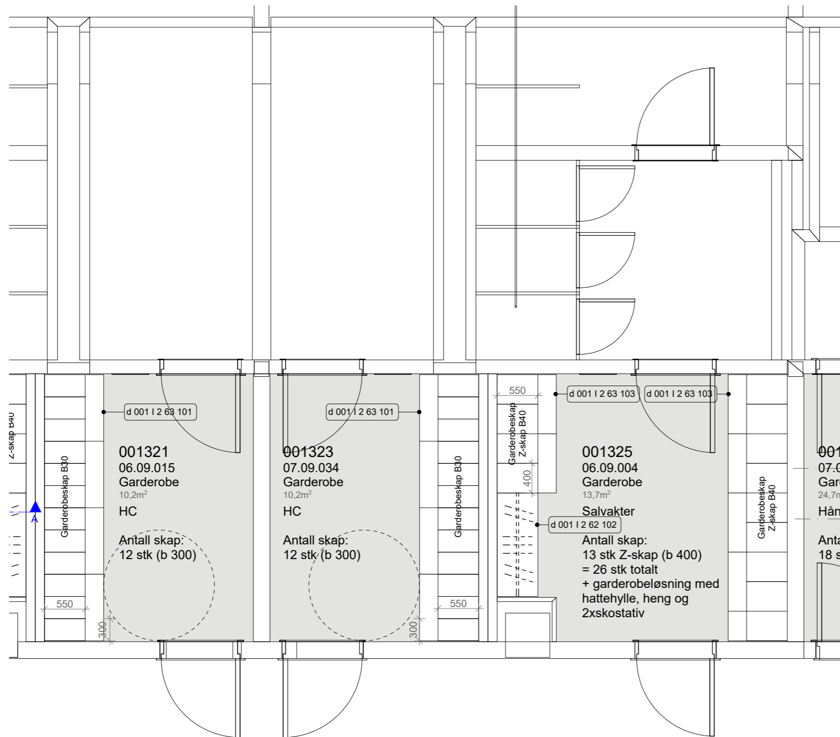
PLAN 1:50
