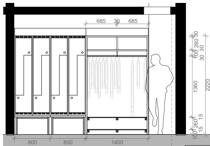
OPPRISS 001 | 2 63 103.B 1:50
