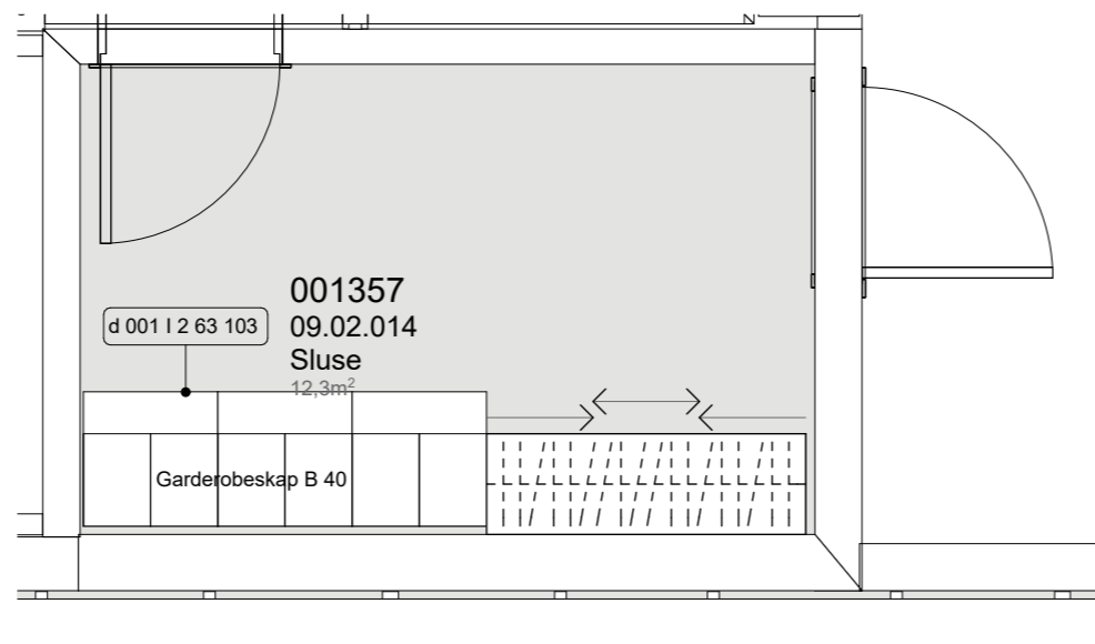
PLAN 1:50
