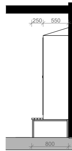
OPPRISS 001 | 2 63 101.C 1:50
