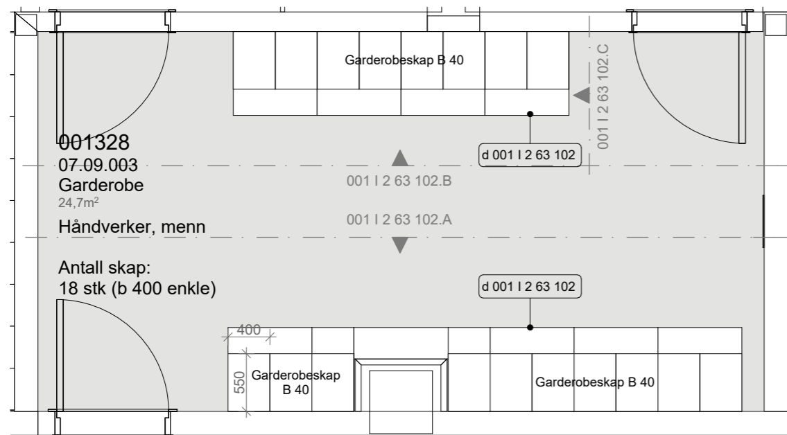
PLAN 1:50
