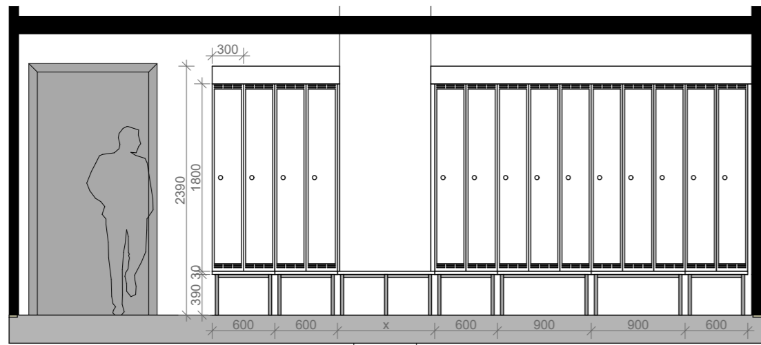
OPPRISS 001 | 2 63 101.A 1:50
