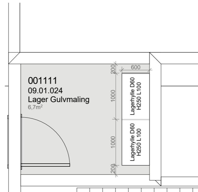
PLAN 1:50
