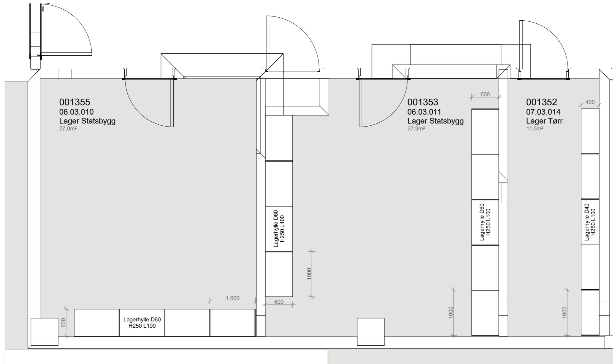
PLAN 1:50
