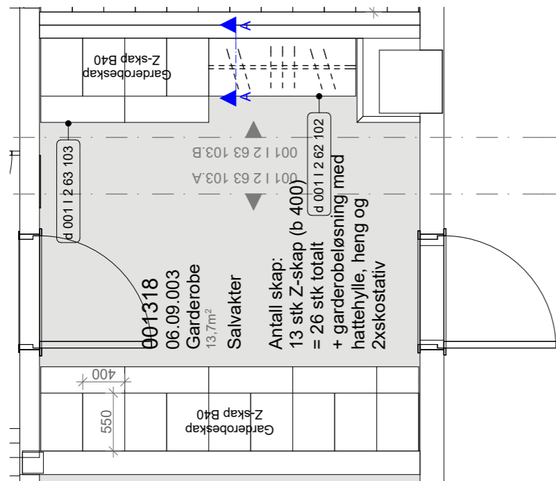
PLAN 1:50
