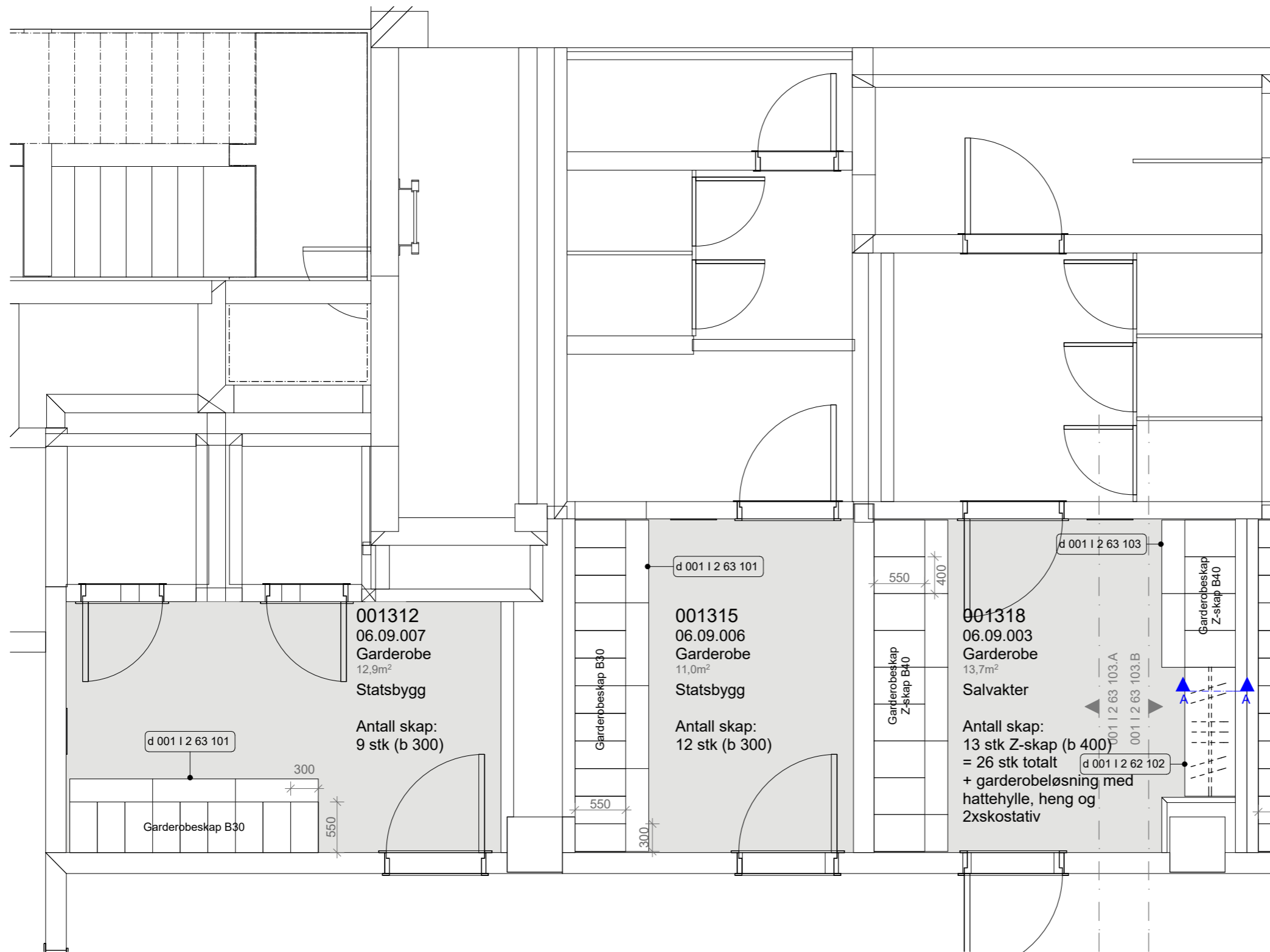
PLAN 1:50
