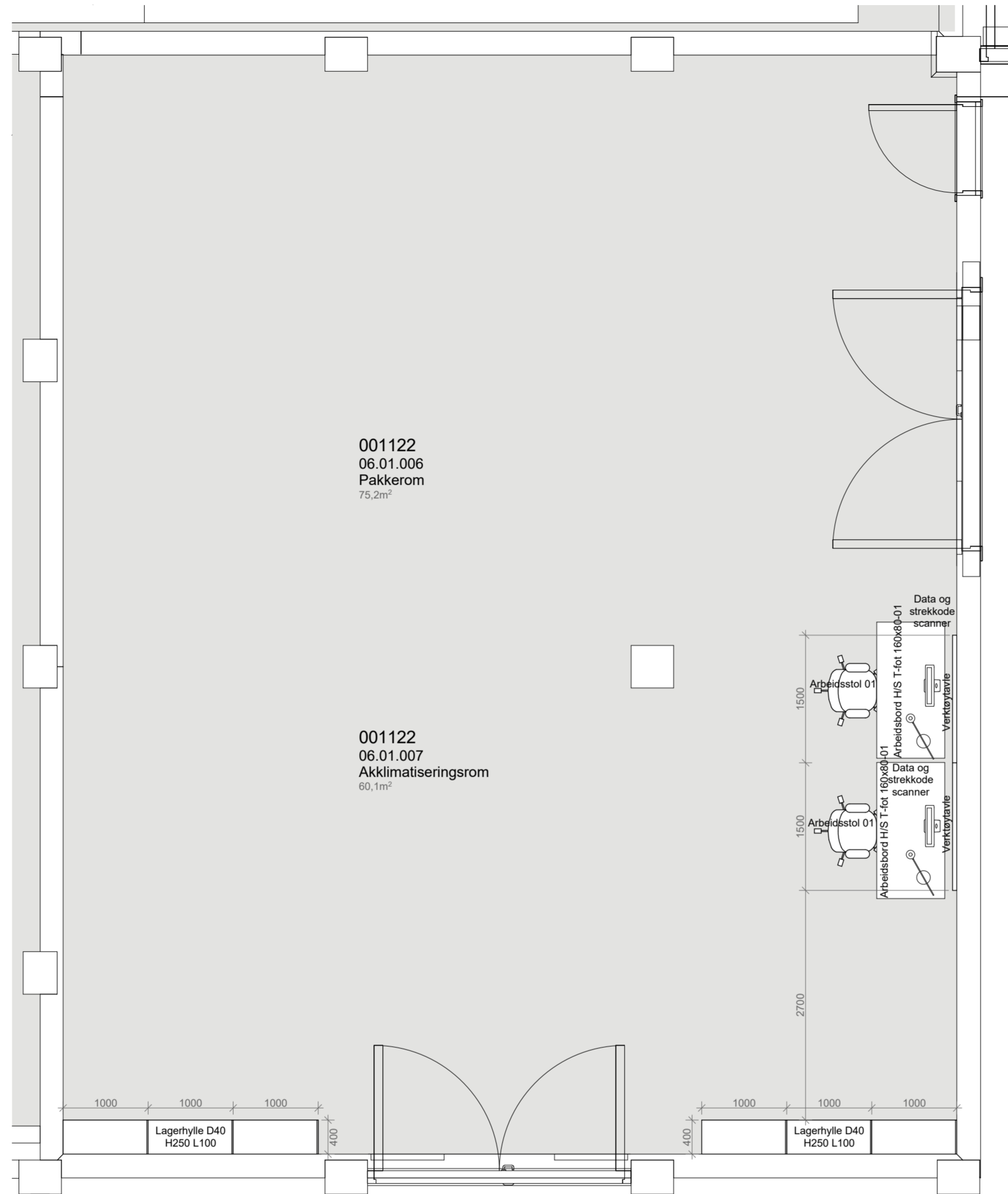
PLAN 1:50
