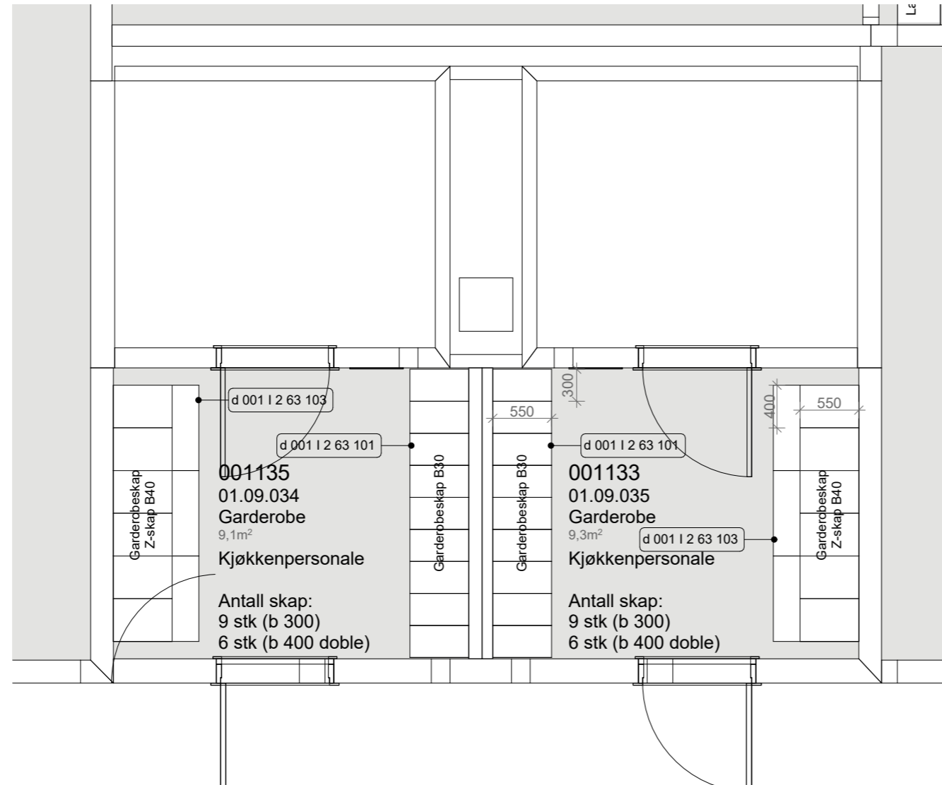
PLAN 1:50
