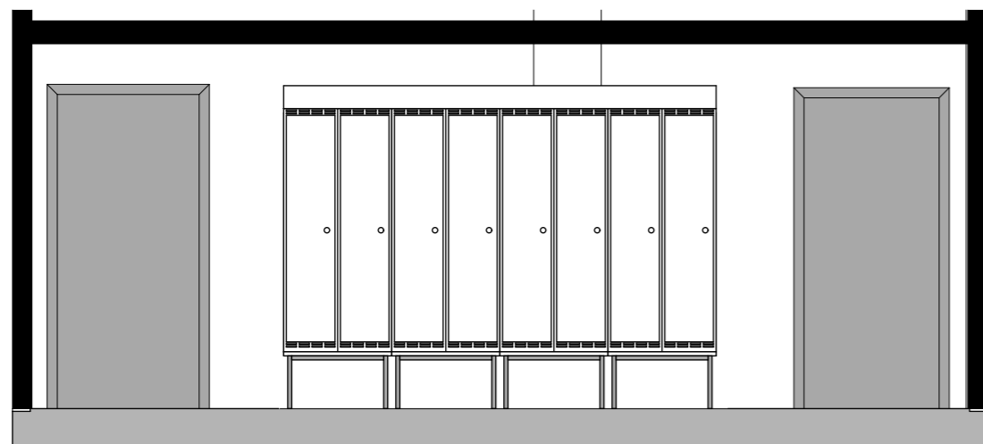
OPPRISS 001 | 2 63 102.B 1:50
