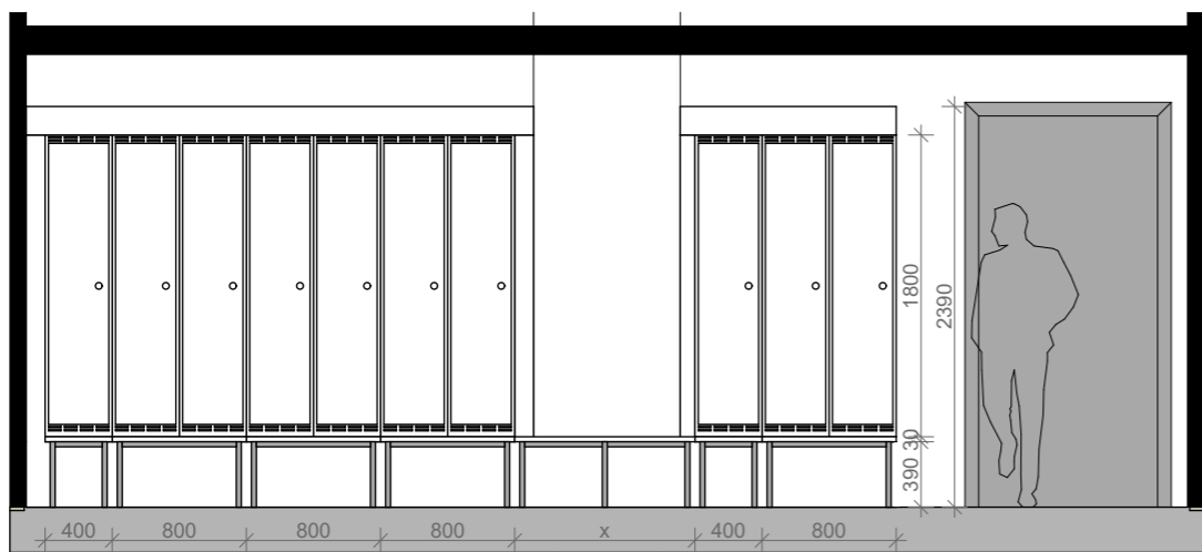
OPPRISS 001 | 2 63 102.A 1:50
