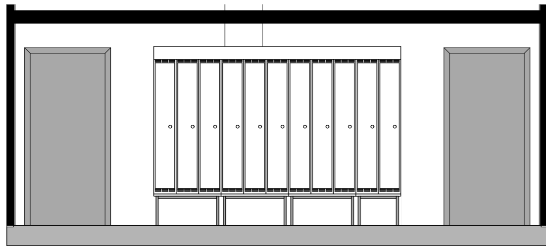
OPPRISS 001 | 2 63 101.B 1:50
