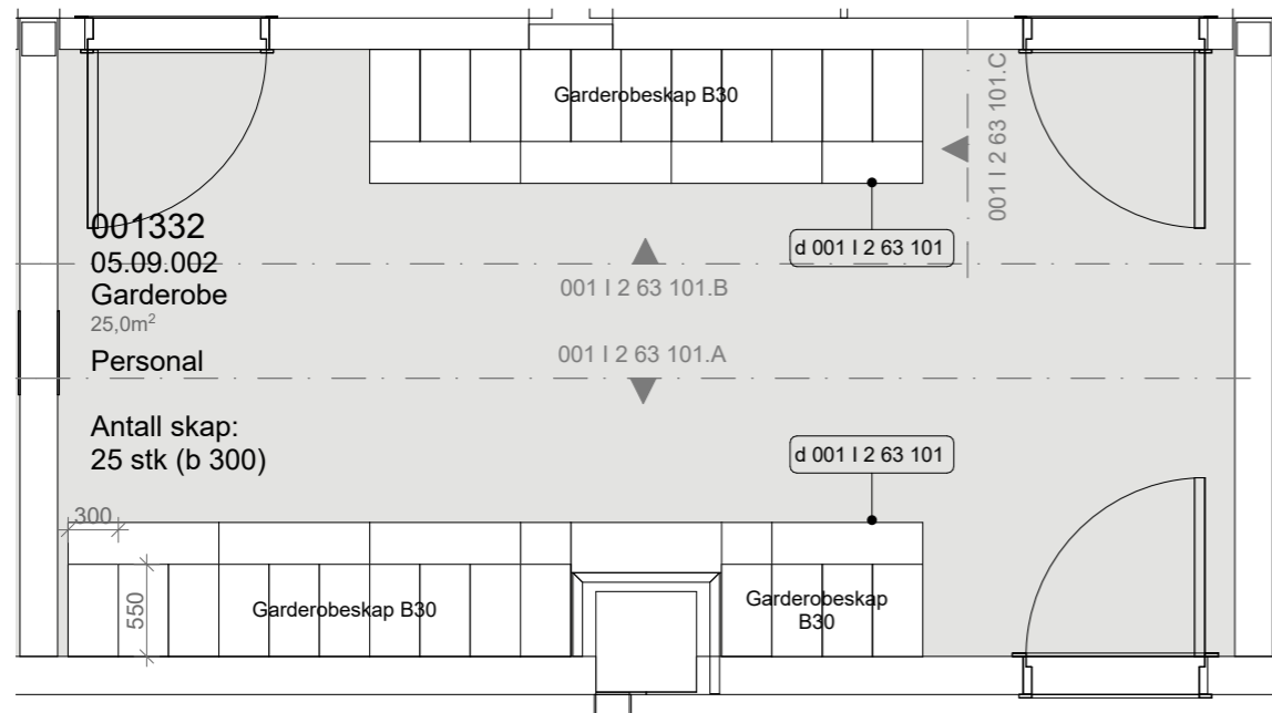
PLAN 1:50
