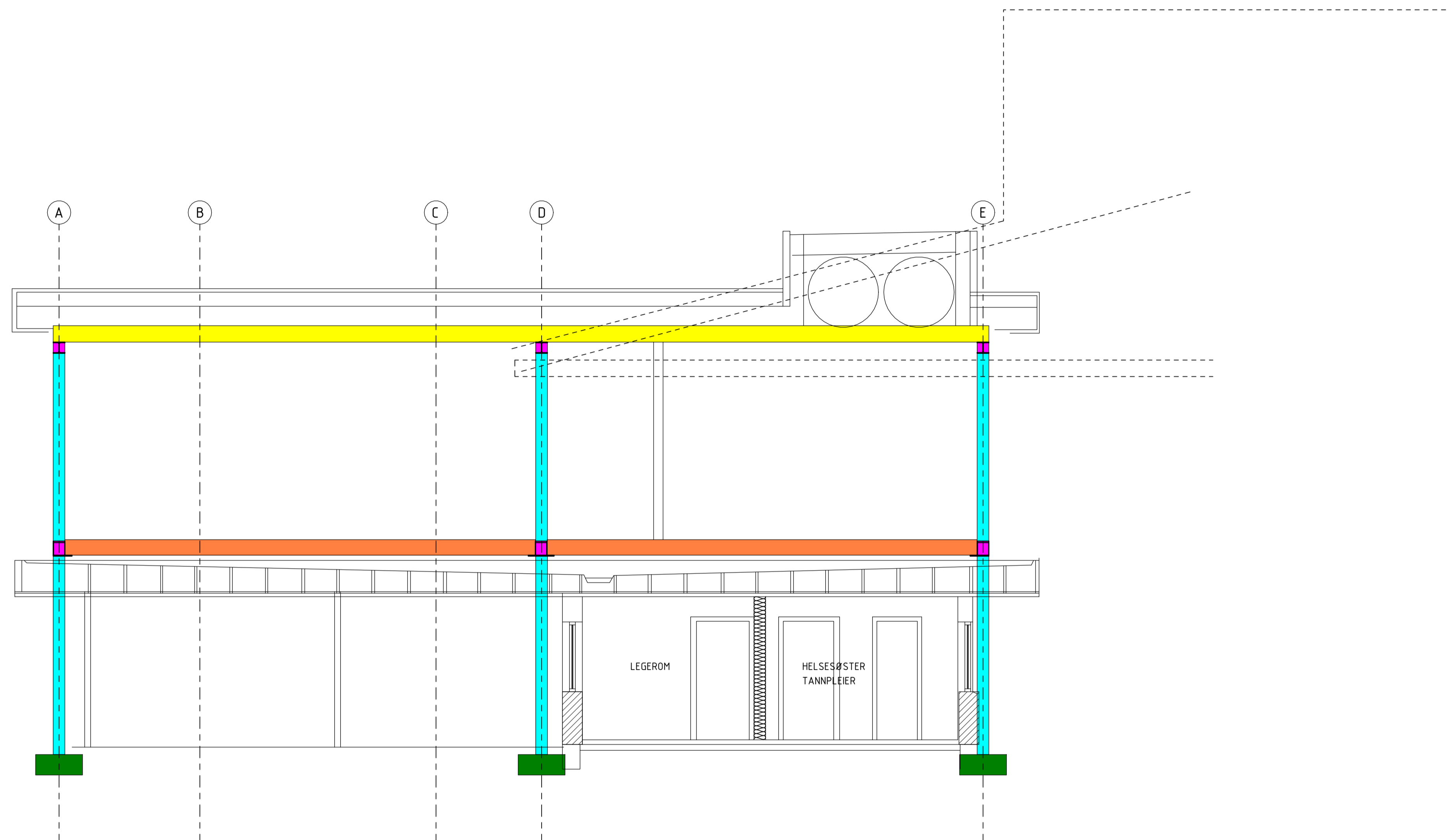
Snitt B-B 1 : 50
