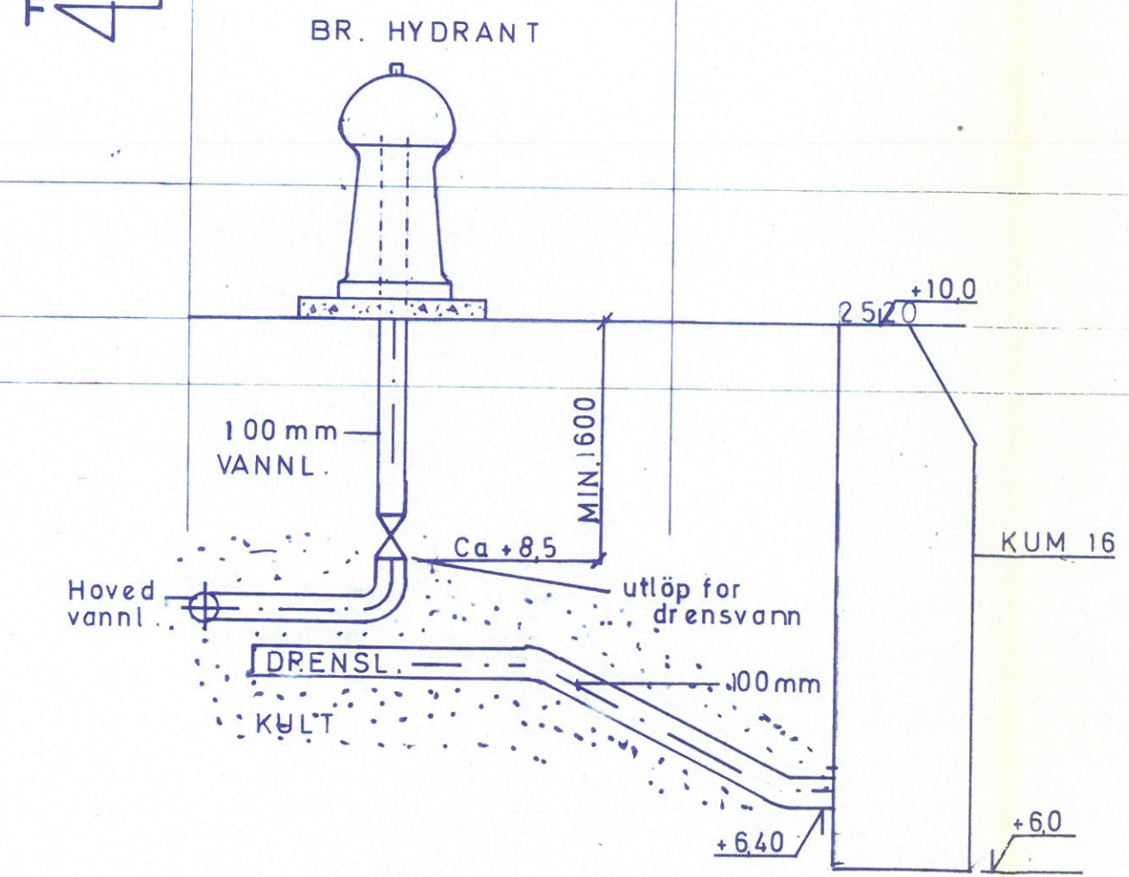
DETALJ AV BR. HYDR. M/RÖR H= 1:50
