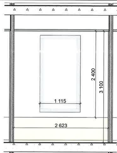
OPPRISS VINDU FASADE TYPE 1
