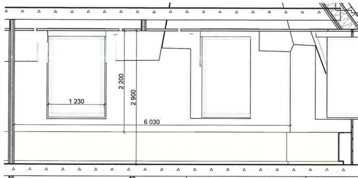
OPPRISS VINDU FASADE TYPE 4
