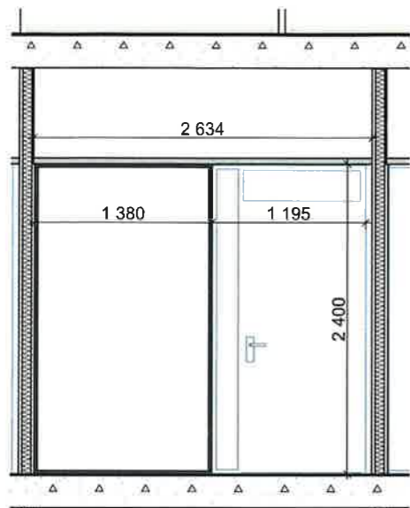
OPPRISS INNVEDIG GLASSFELT TYPE A
