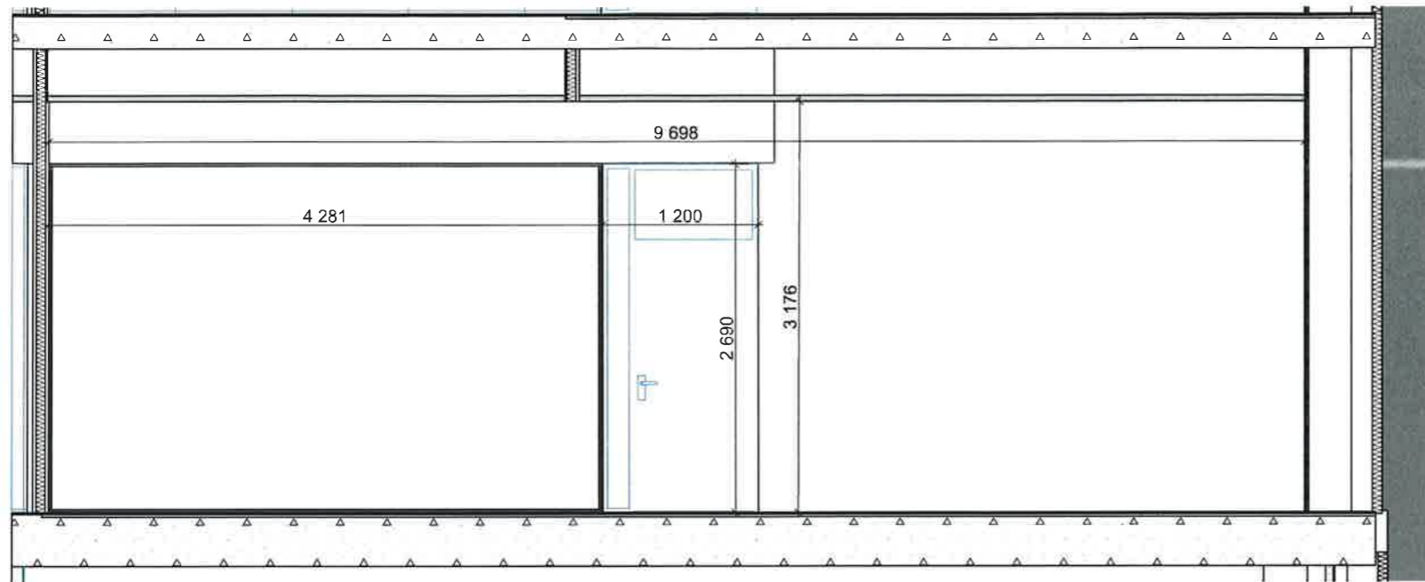
OPPRISS INNVEDIG GLASSFELT TYPE D
