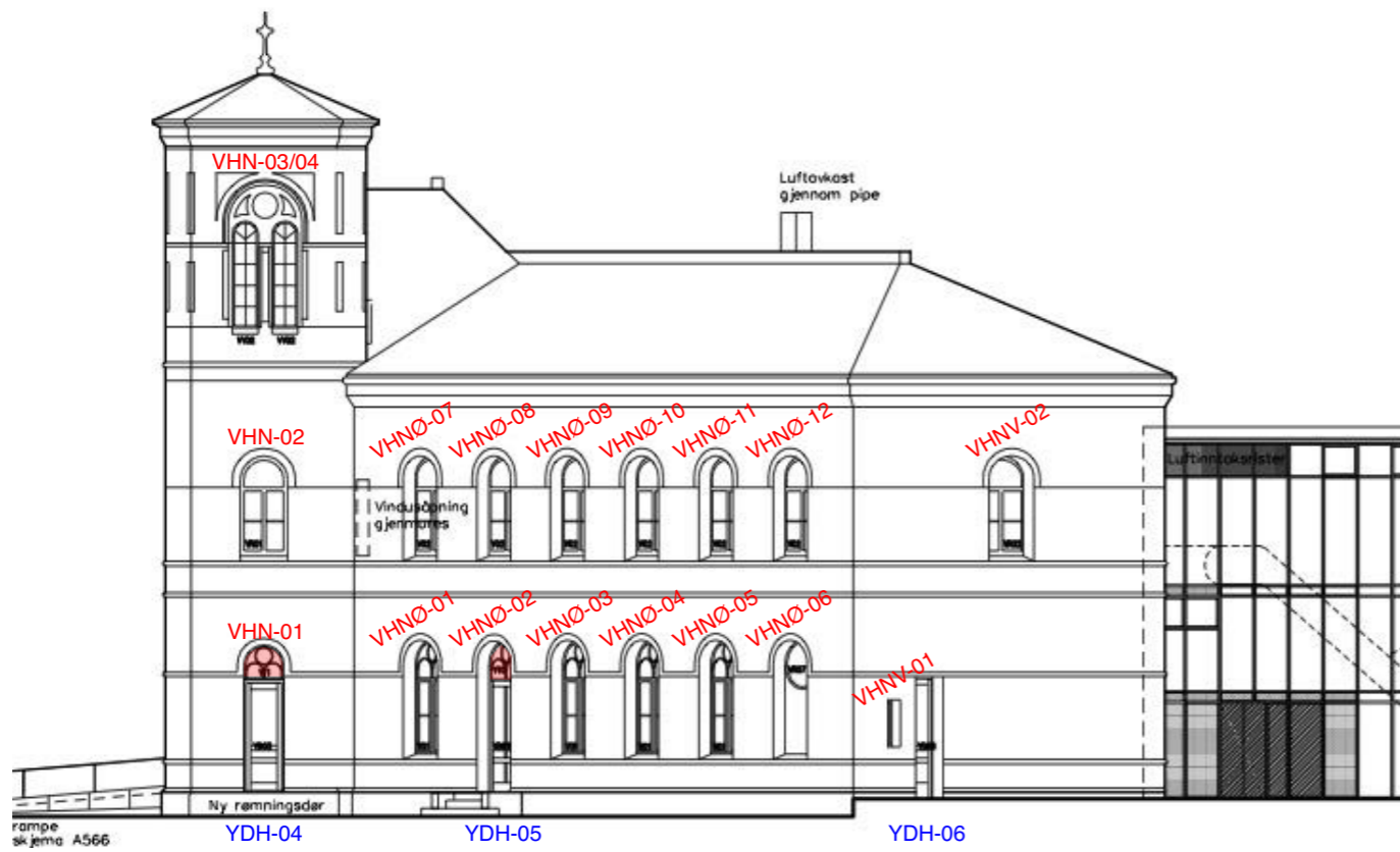
Fasade NORD
