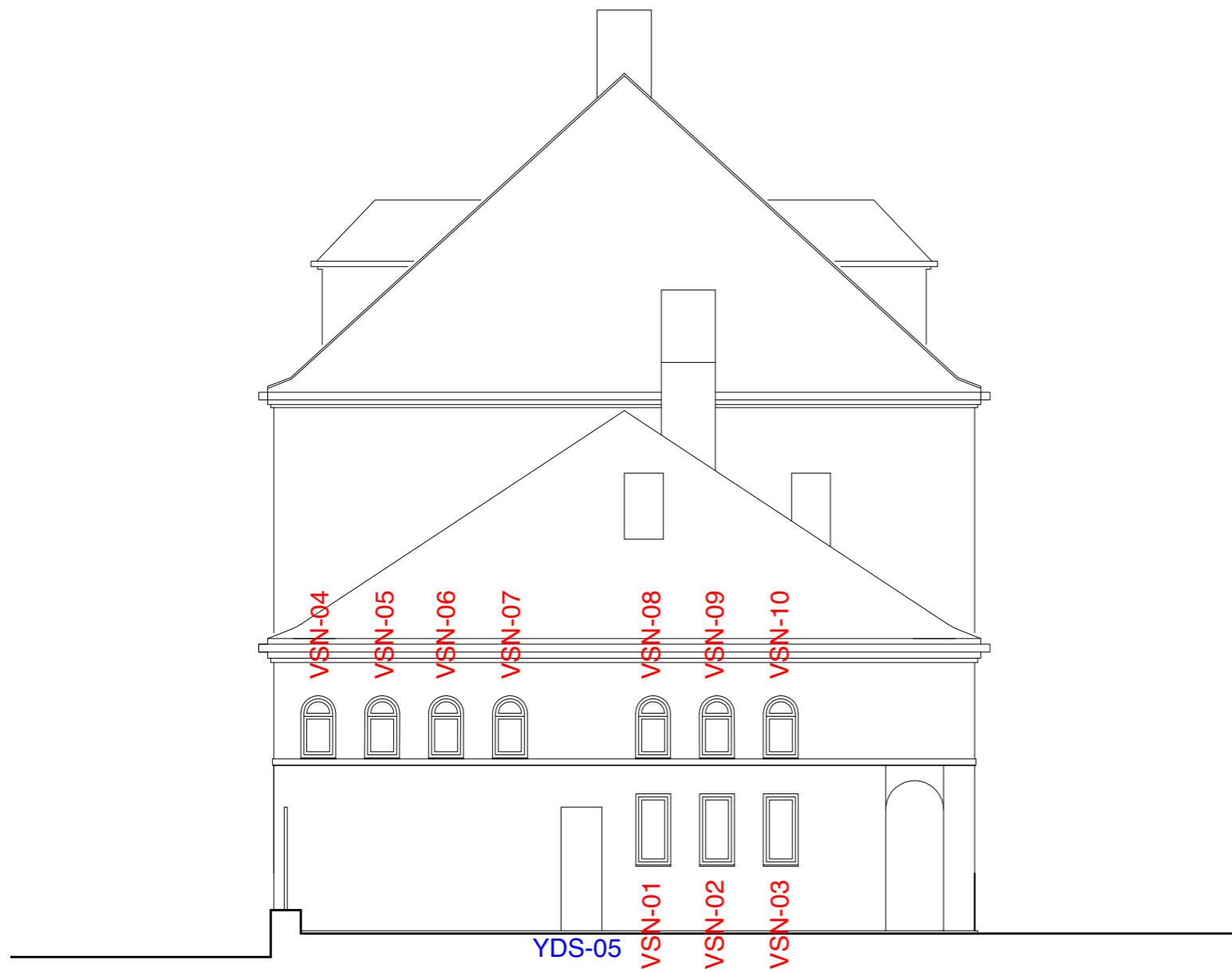
Fasade NORD
