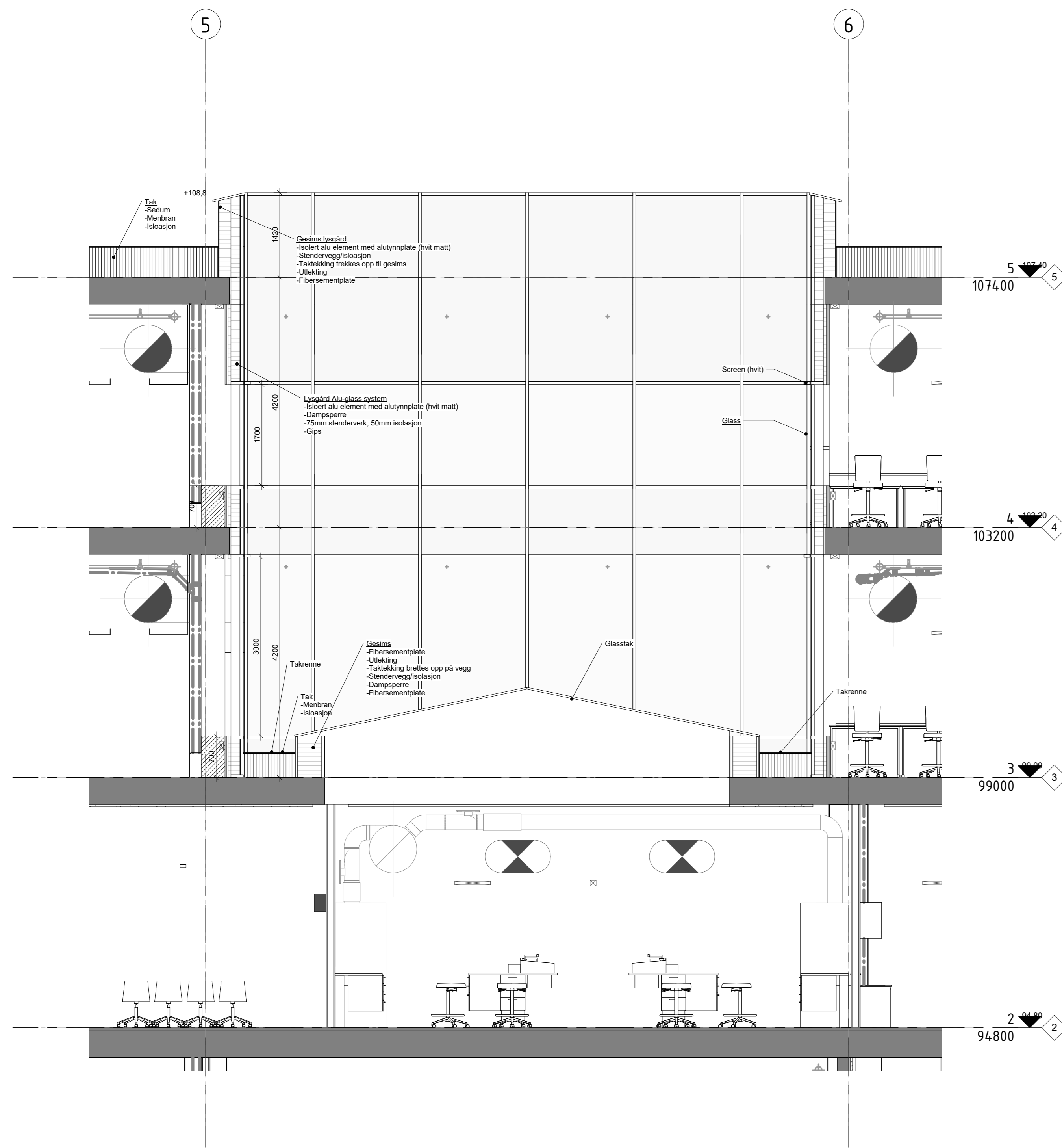
snitt lysgård 4-1
