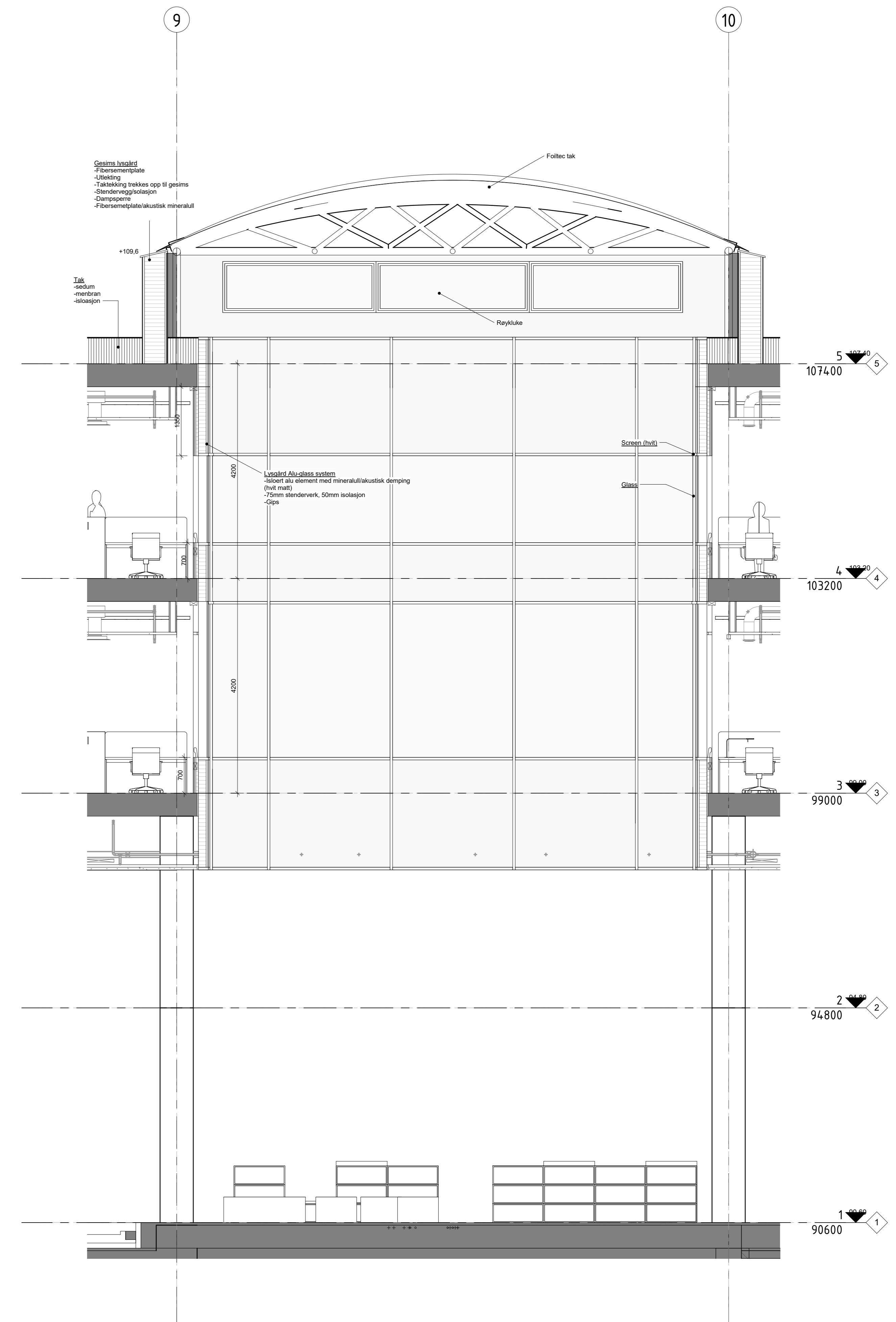
snitt lysgård 4-3
