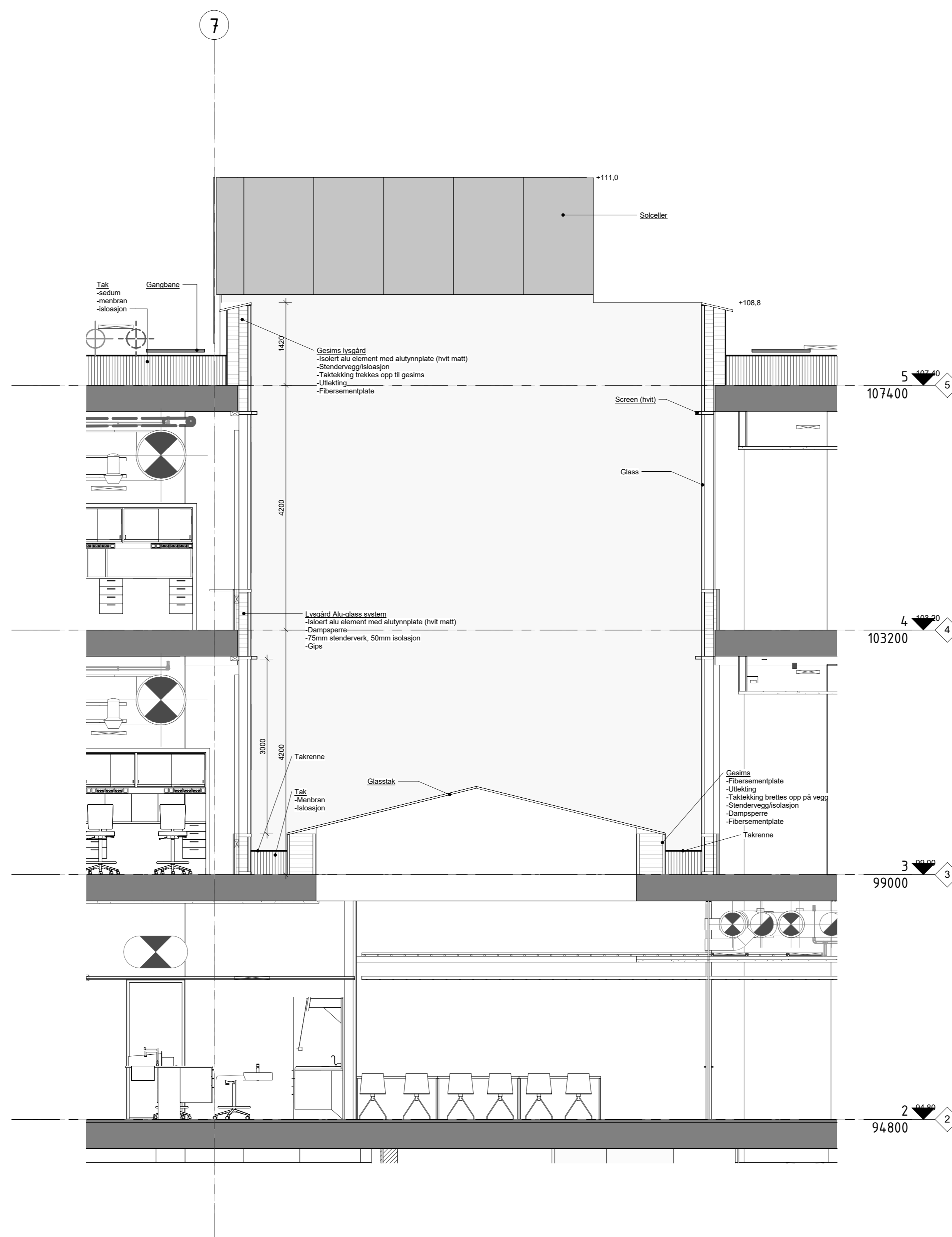
snitt lysgård 4-2
