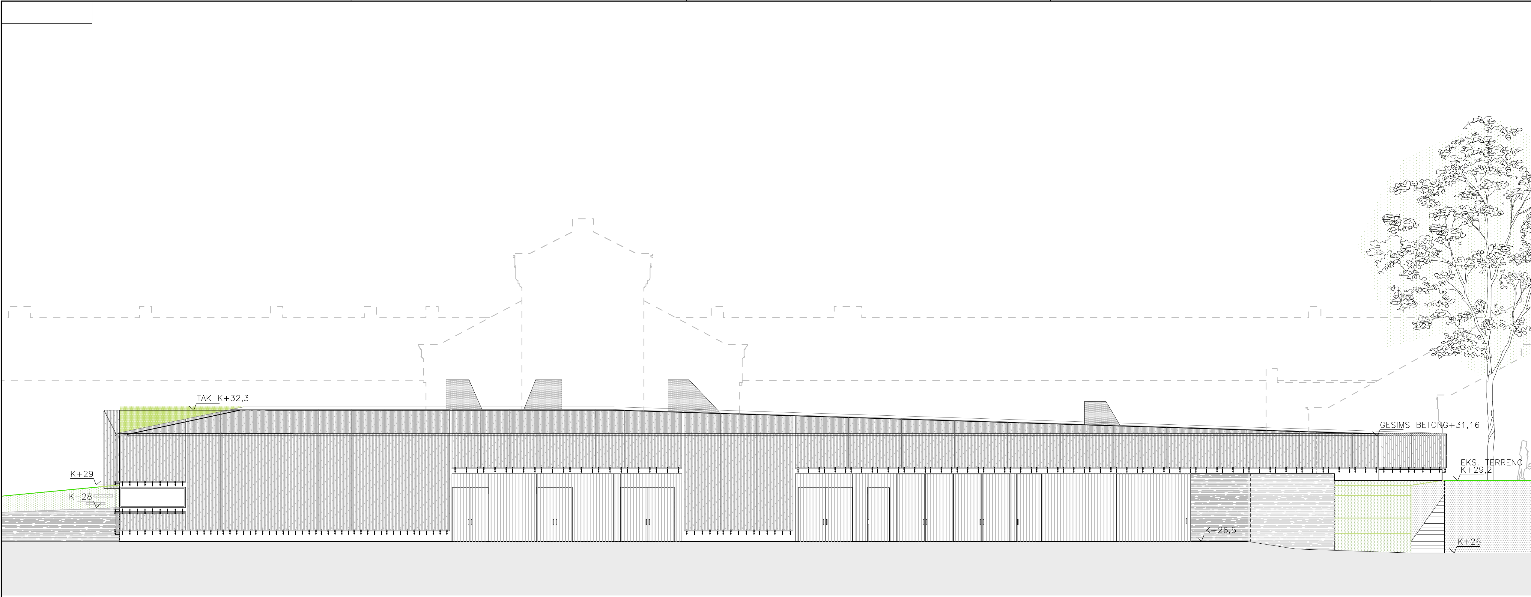
FASADE VEST
