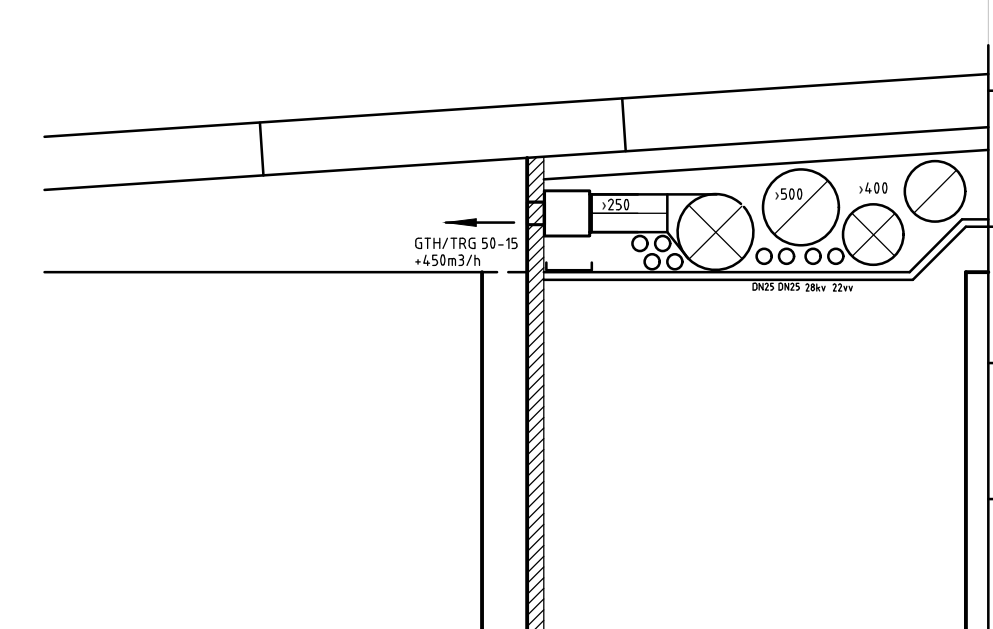
Snitt A-A
