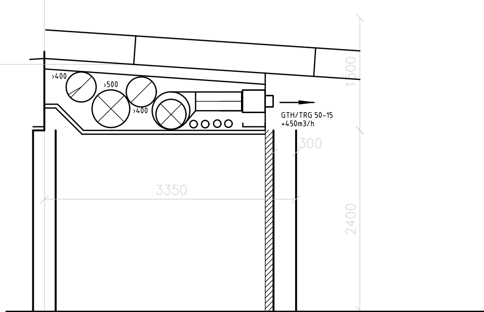
Snitt B-B
