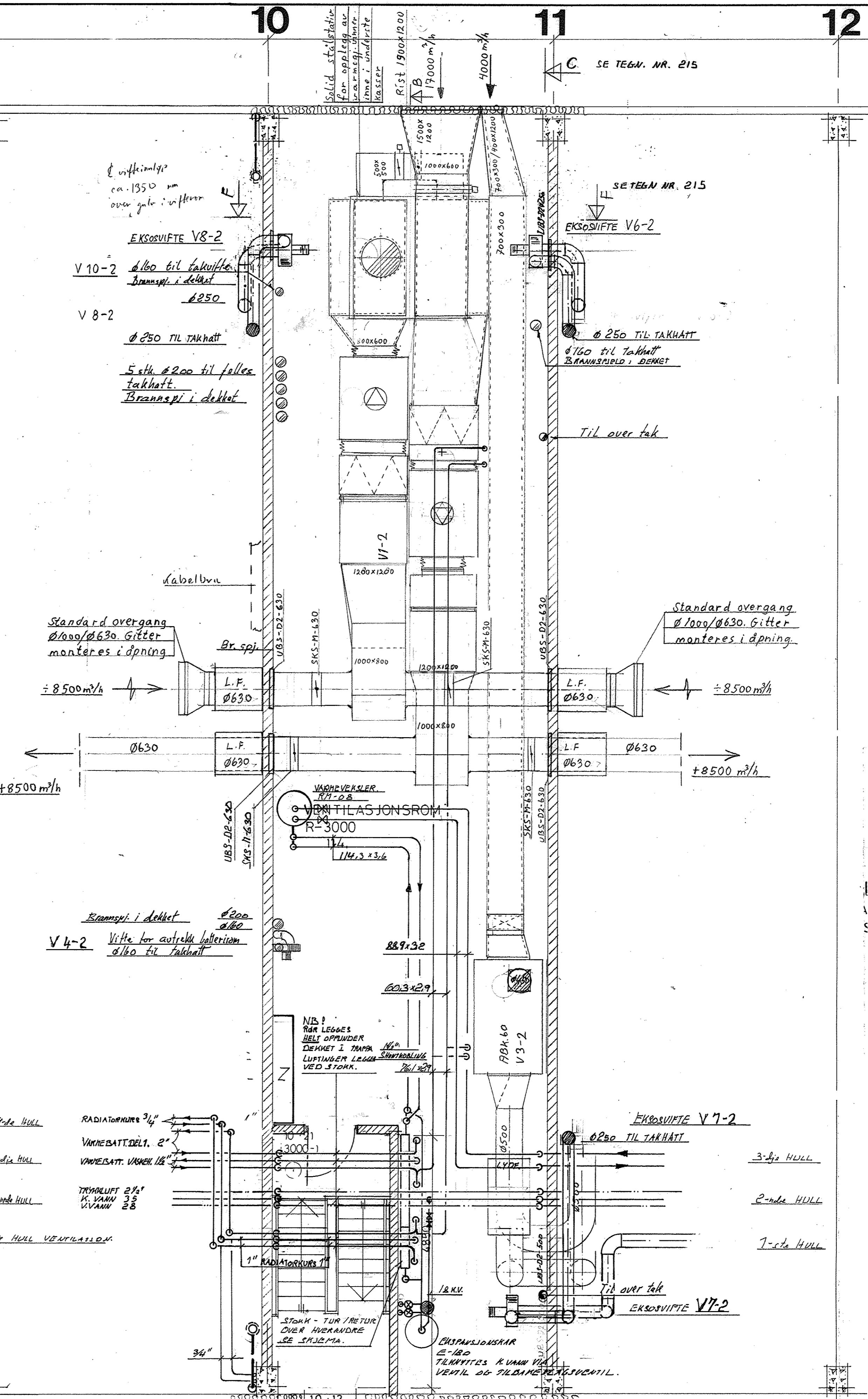
PLAN 3 ETASJE (MEZZANIN) MELLOM AKSE 10 OG 11
