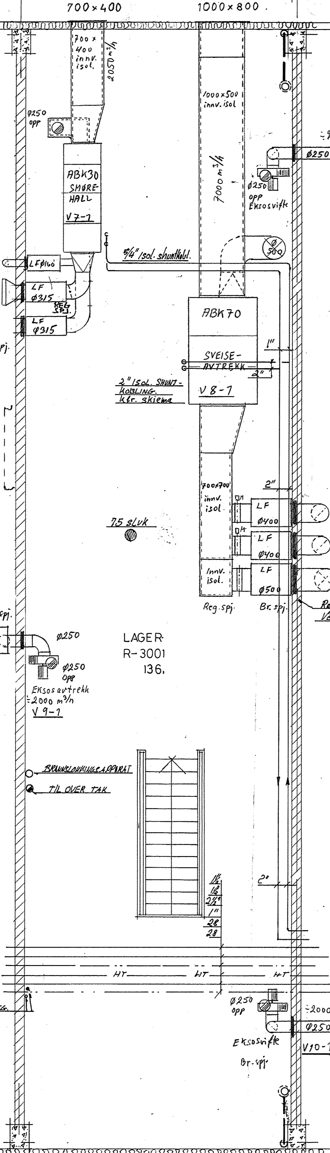
PLAN 3 ETASJE (MEZZANIN) MELLOM AKSE 3 OG 4.
