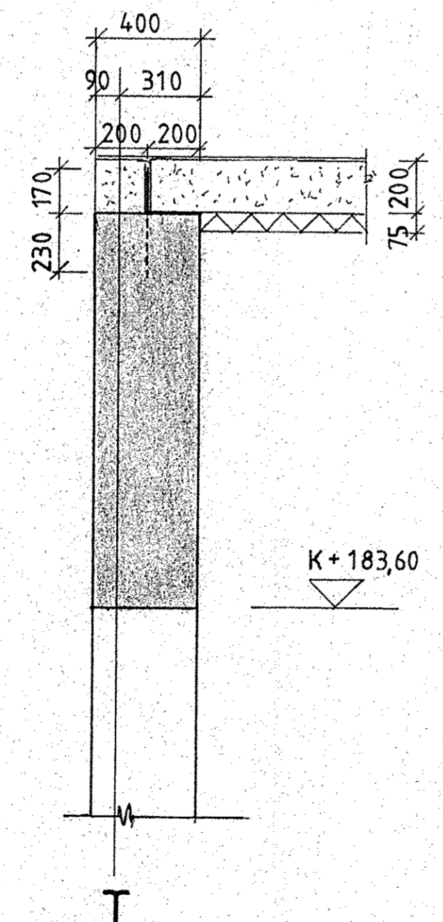
SNITT A-A 1:20
