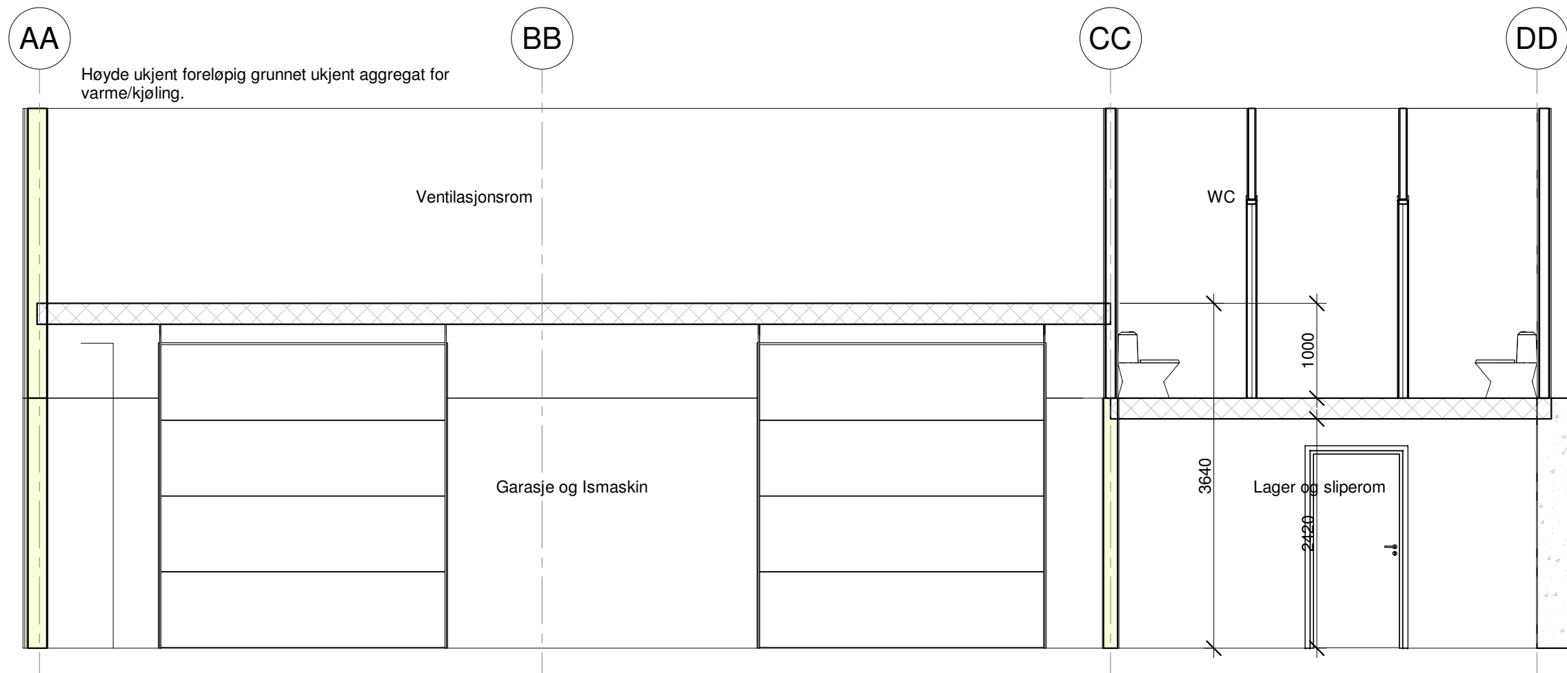
Utsnitt av snitt påbygg Høydeforsjell i Akse CC
