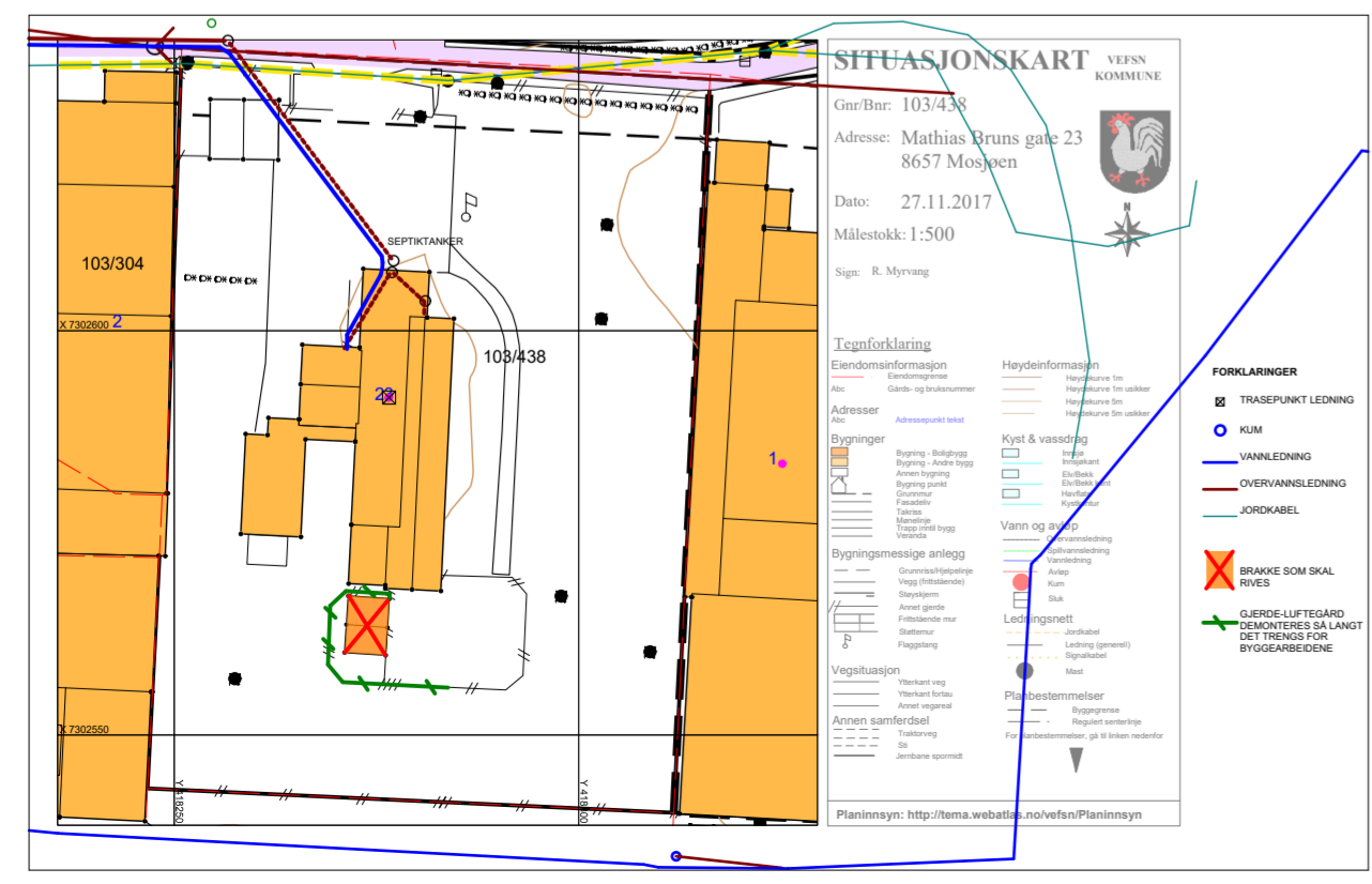
SITUASJONSKART 1:1000
