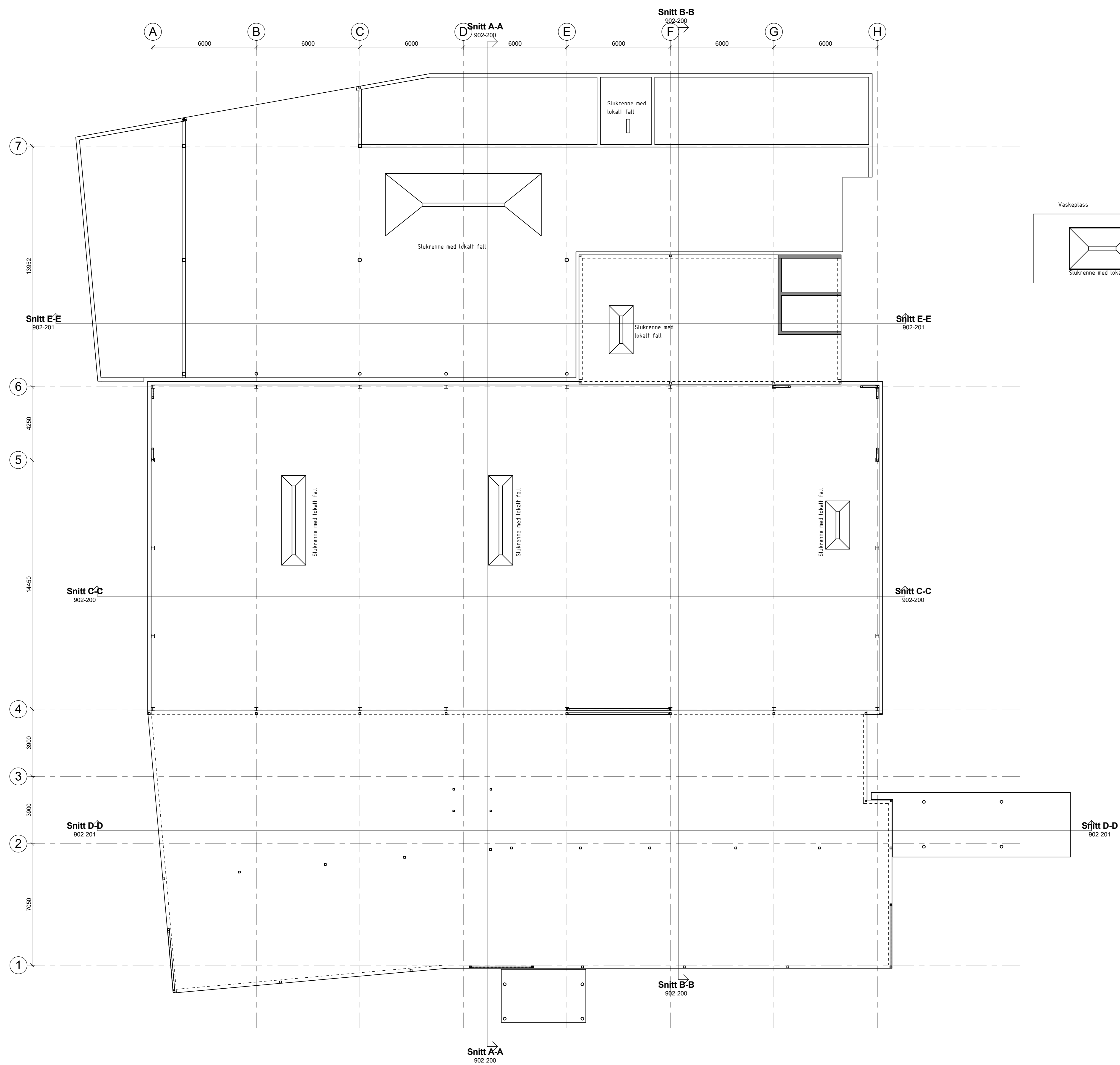
Plan 1. etasje 1 : 100
