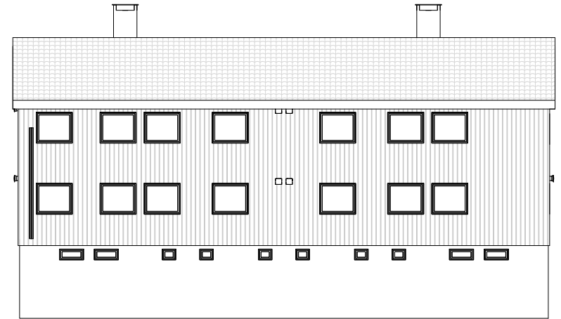
Vest 1 : 200
