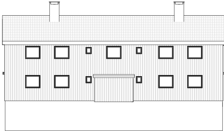
Nord 1 : 200
