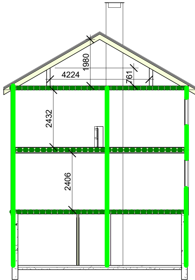
Snitt 1 Brann 1 : 100
