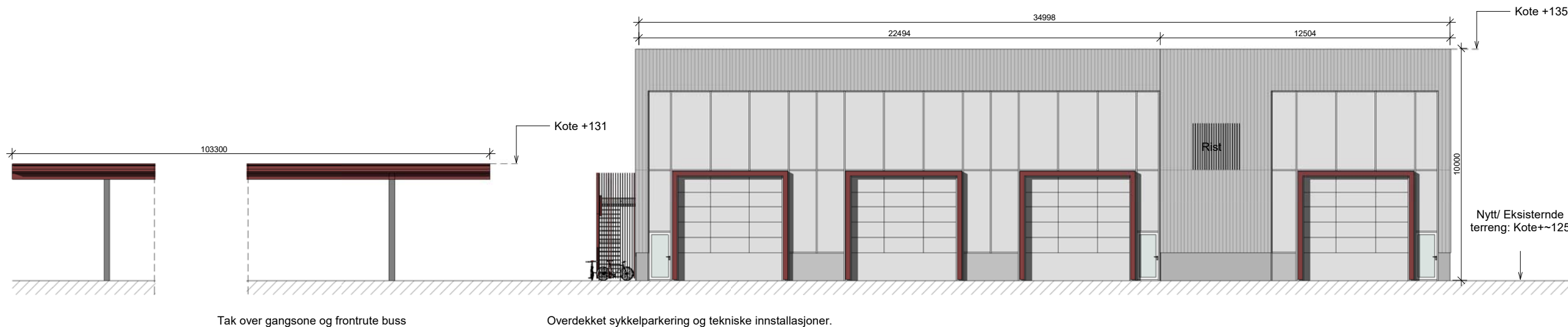
Fasade Nord 1 : 100
