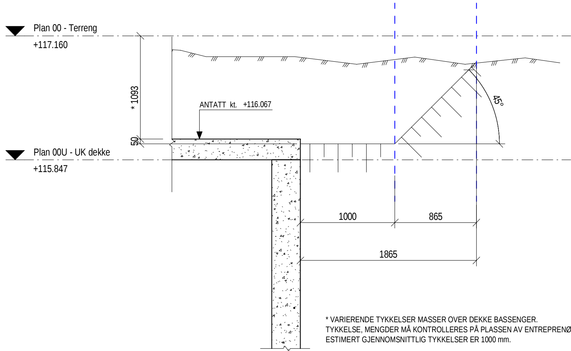
PRINSIPP GRAVESKRÅNING 1 : 25
