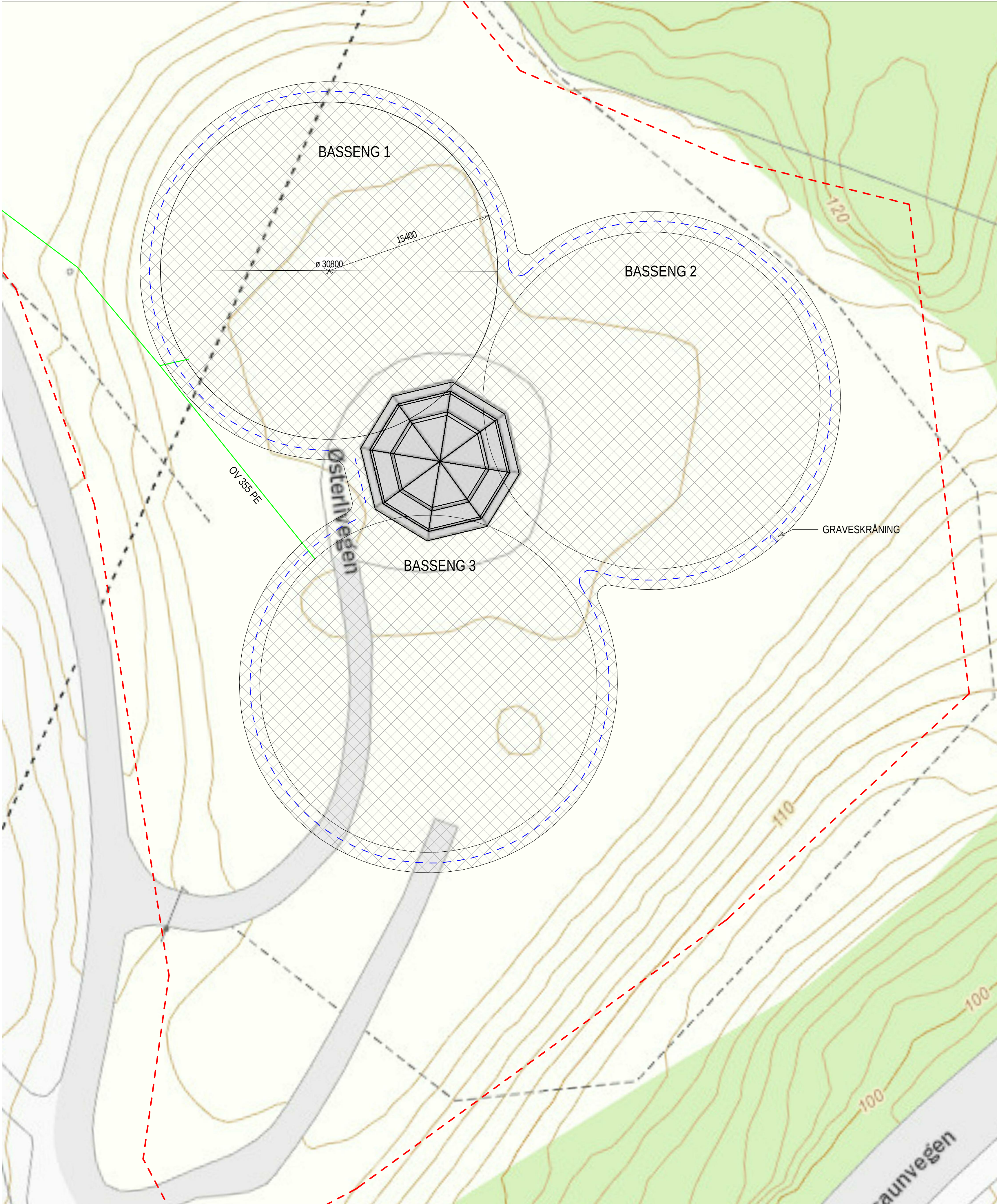
PLAN 1 : 200
