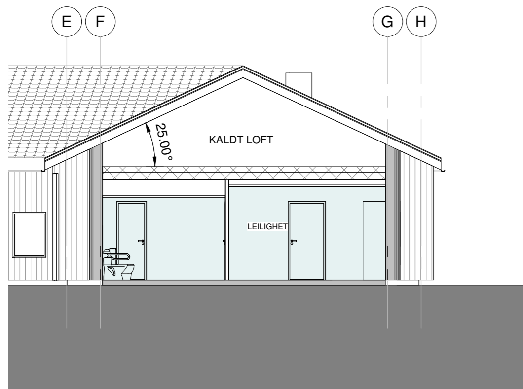
1 AA 1 : 100
