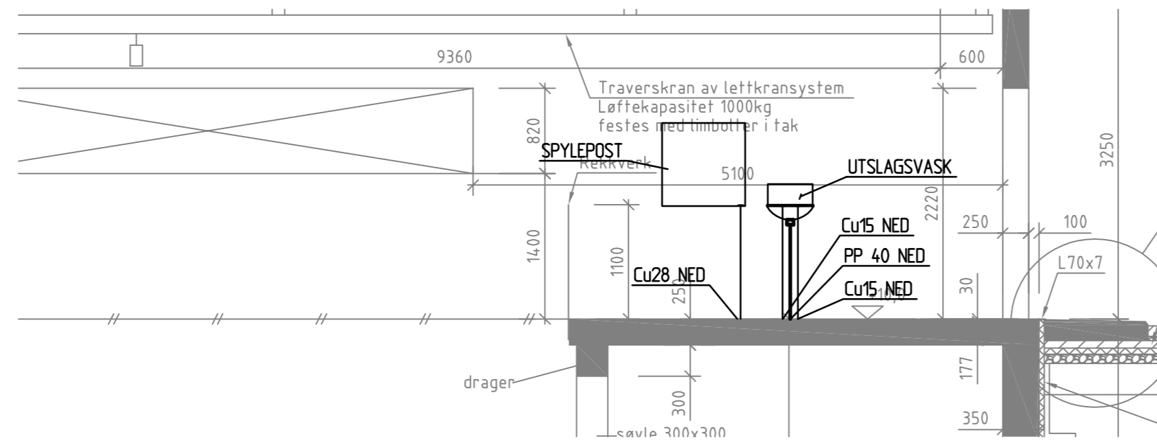
SNITT A-A
