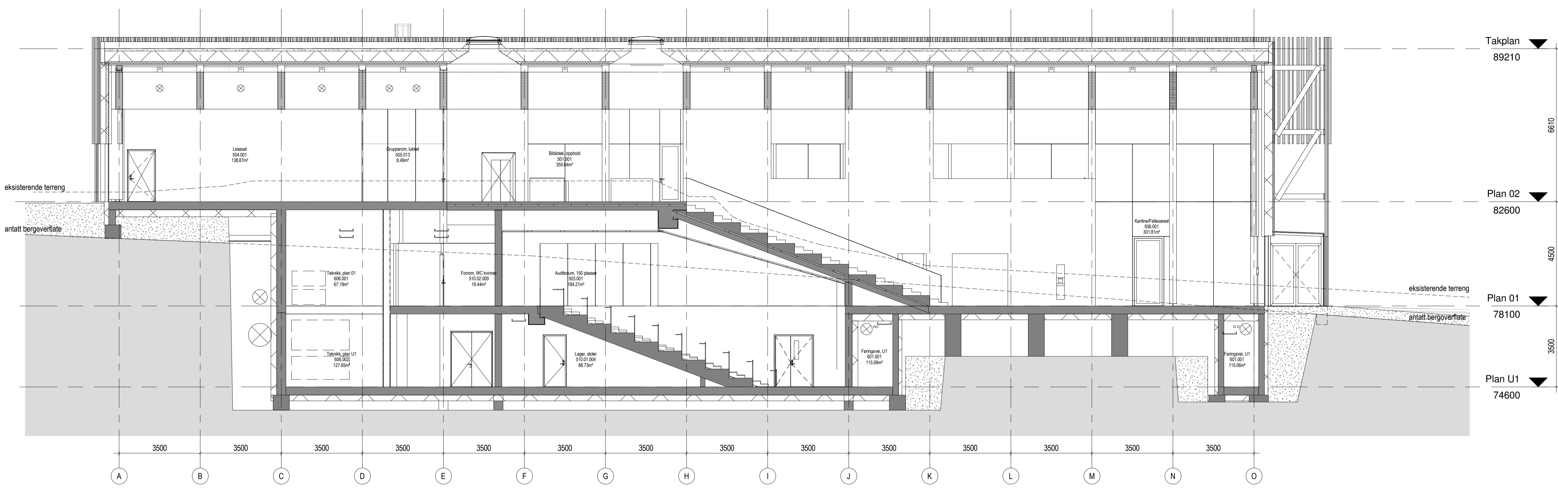
Lengdesnitt 1:100
