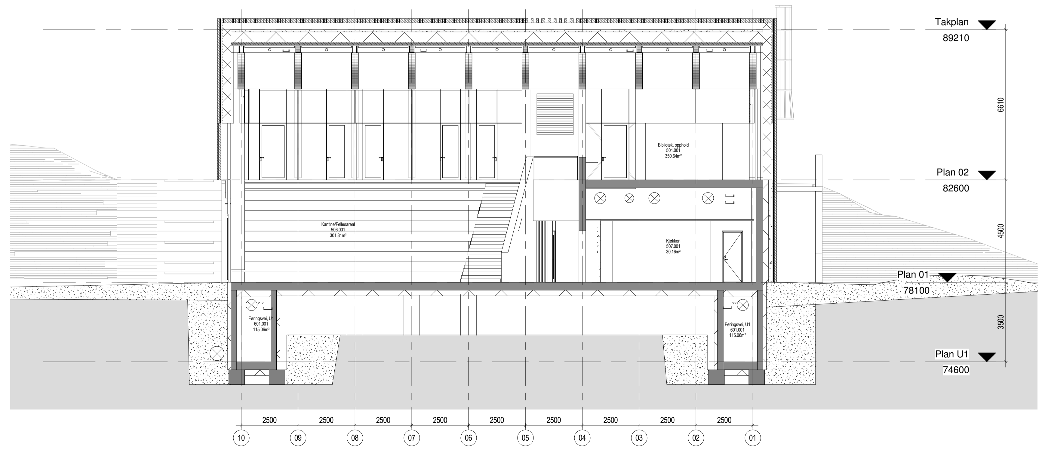
Kortsnitt 1:100
