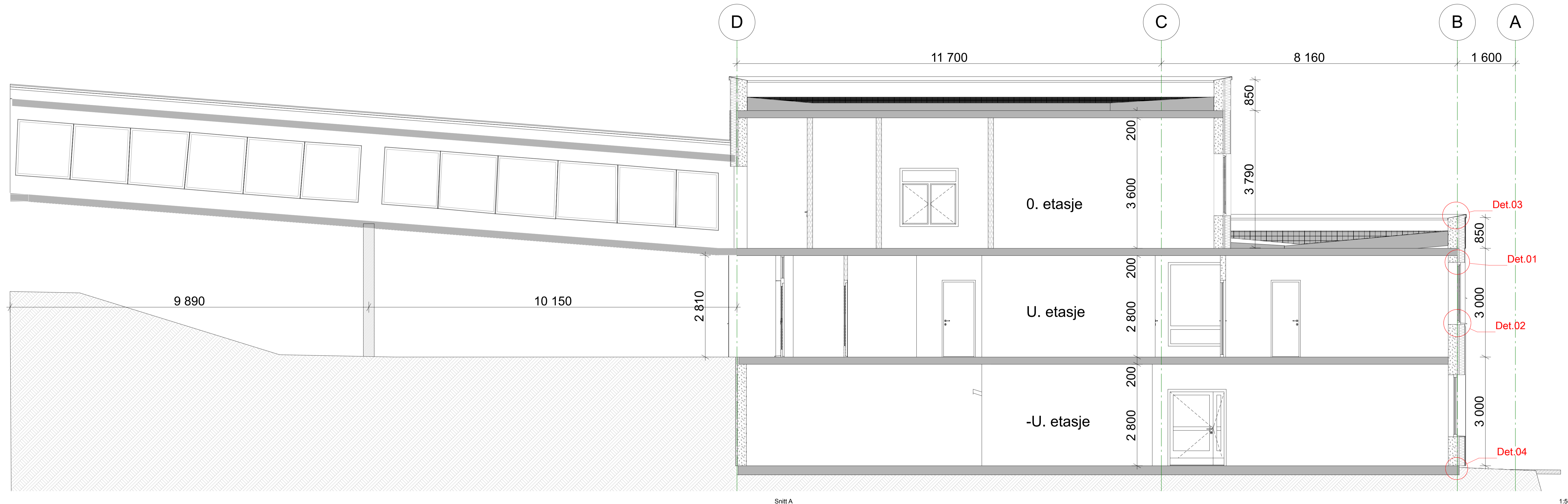
Snitt A
