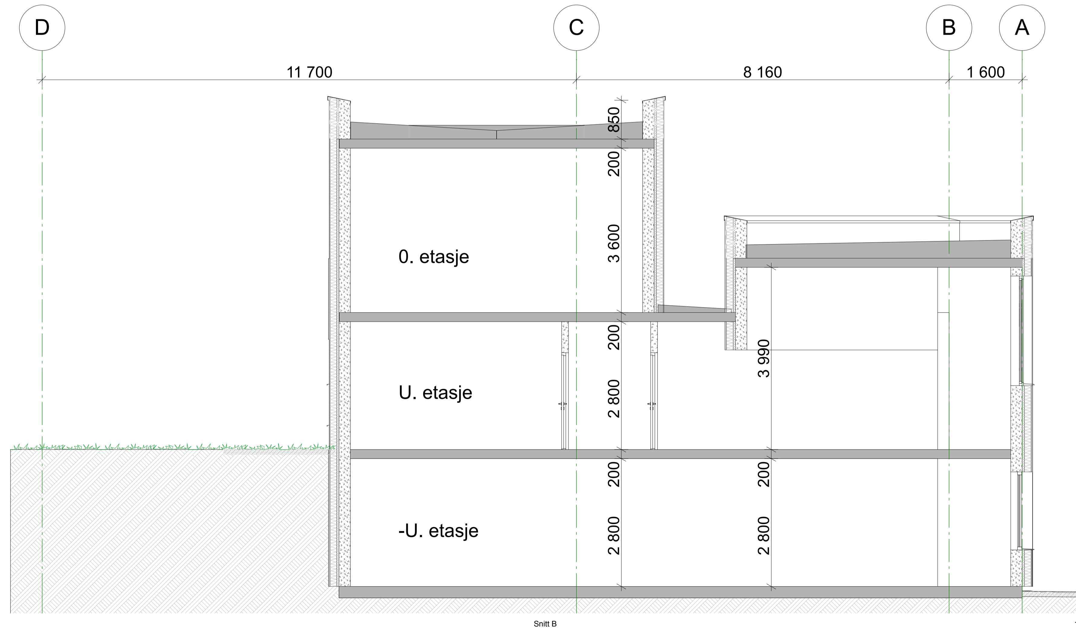
Snitt B
