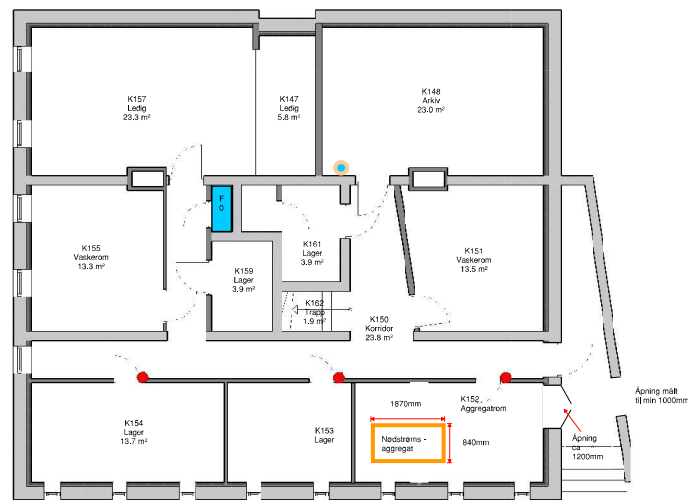
1 Kjeller 1 : 100
