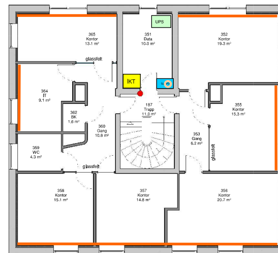
3 Plan 03 1 : 100
