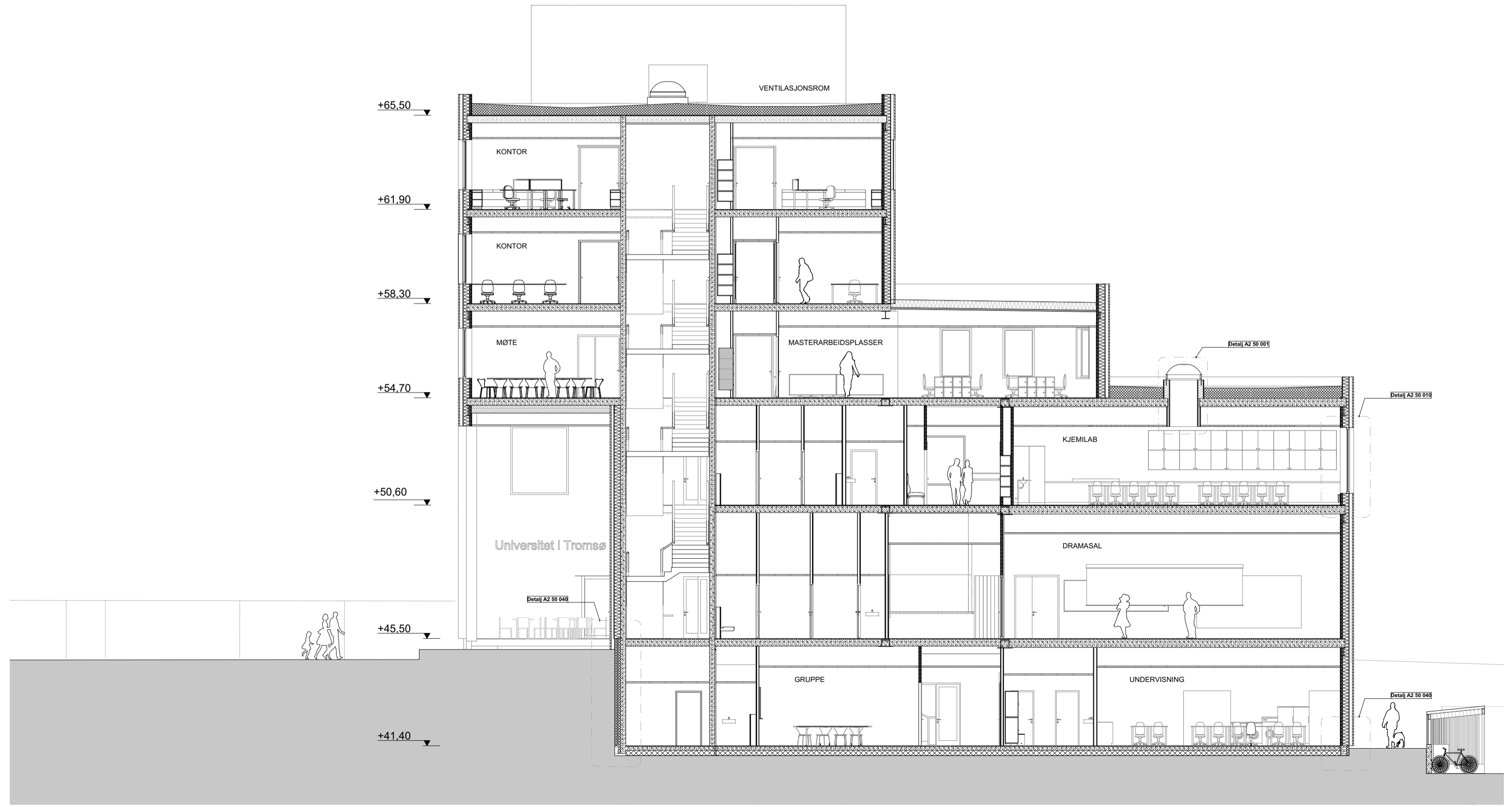
1:125 Snitt B Tversnitt
