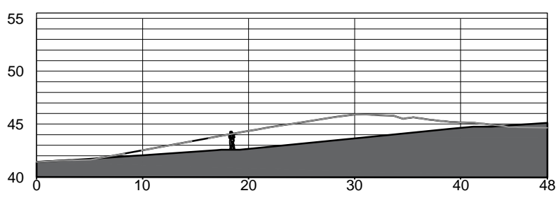
Snittlinje terreng kjøretrasé Snitt A-A
