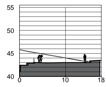
Tversnitt - skråning Snitt B-B
