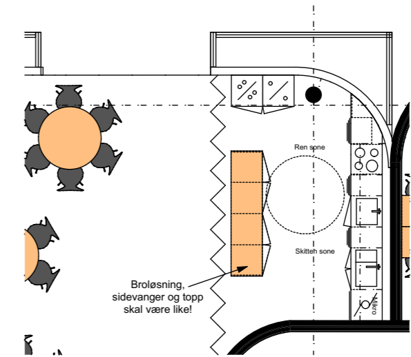
Utsnitt plan 1:100
