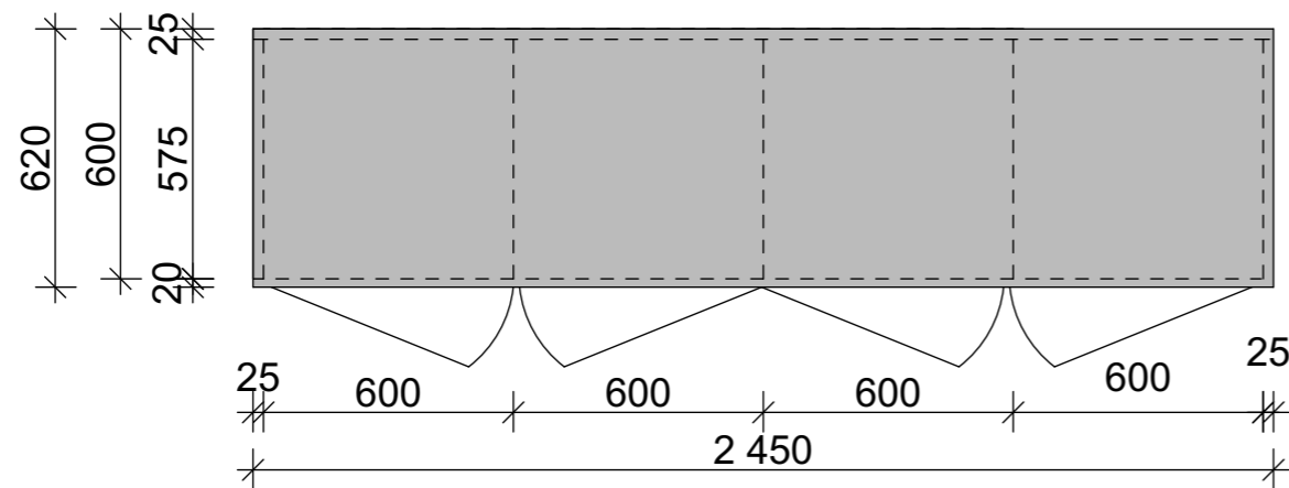
PLAN 1:20
