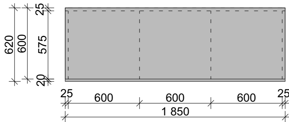
PLAN 1:20
